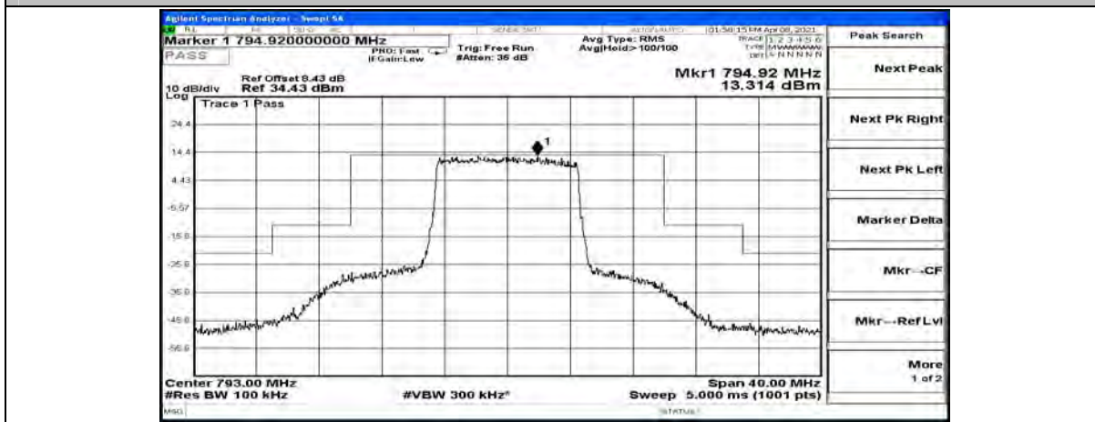
BAND 14_10MHz_QPSK
