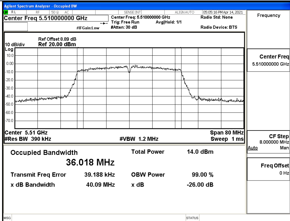
IEEE 802.11ac40 / Channel 102 / 5510MHz
