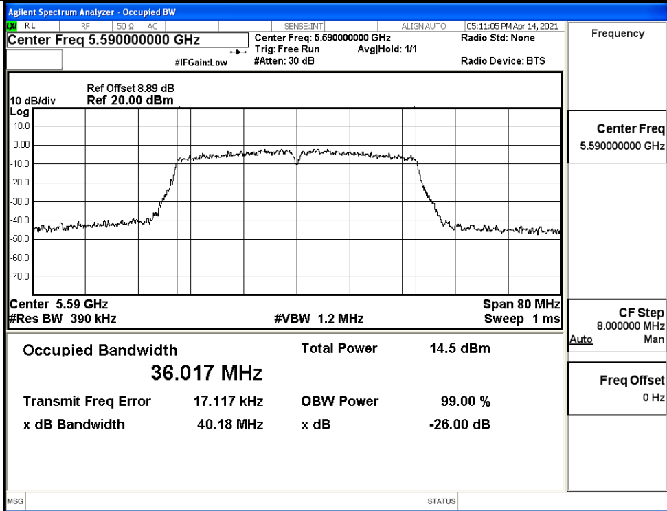
IEEE 802.11ac40 / Channel 118 / 5590MHz
