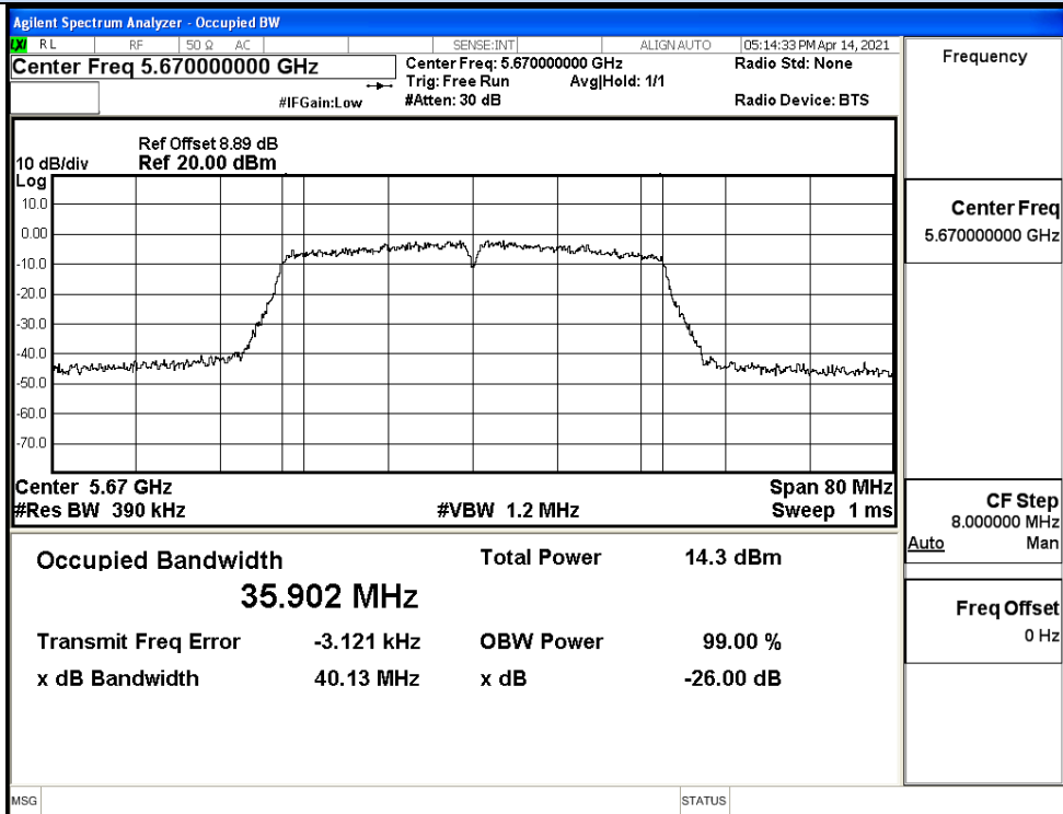
IEEE 802.11ac40 / Channel 134 / 5670MHz
