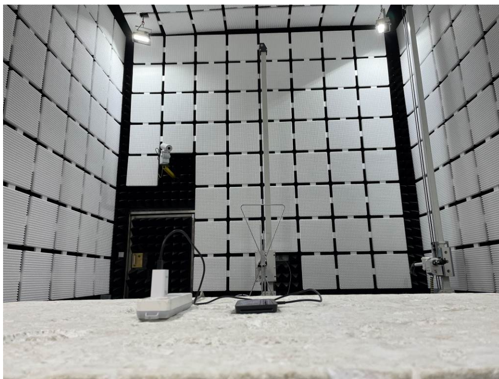
Fig. 2 (30MHz~1GHz)
