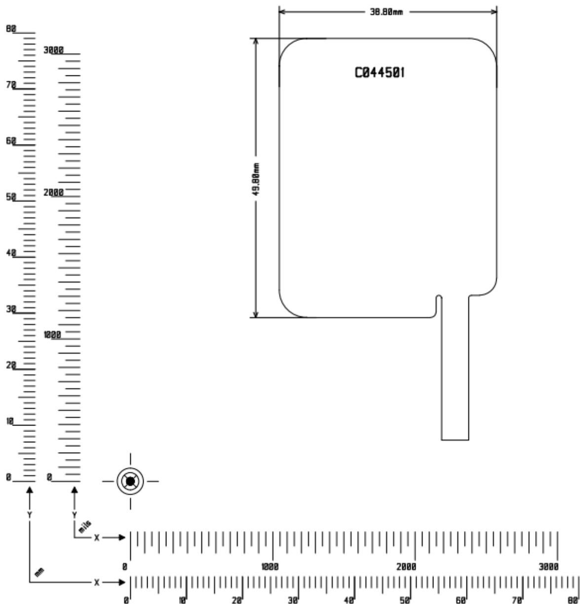
Fig. 4.1.3.1 RFID Antenna Dimensions
