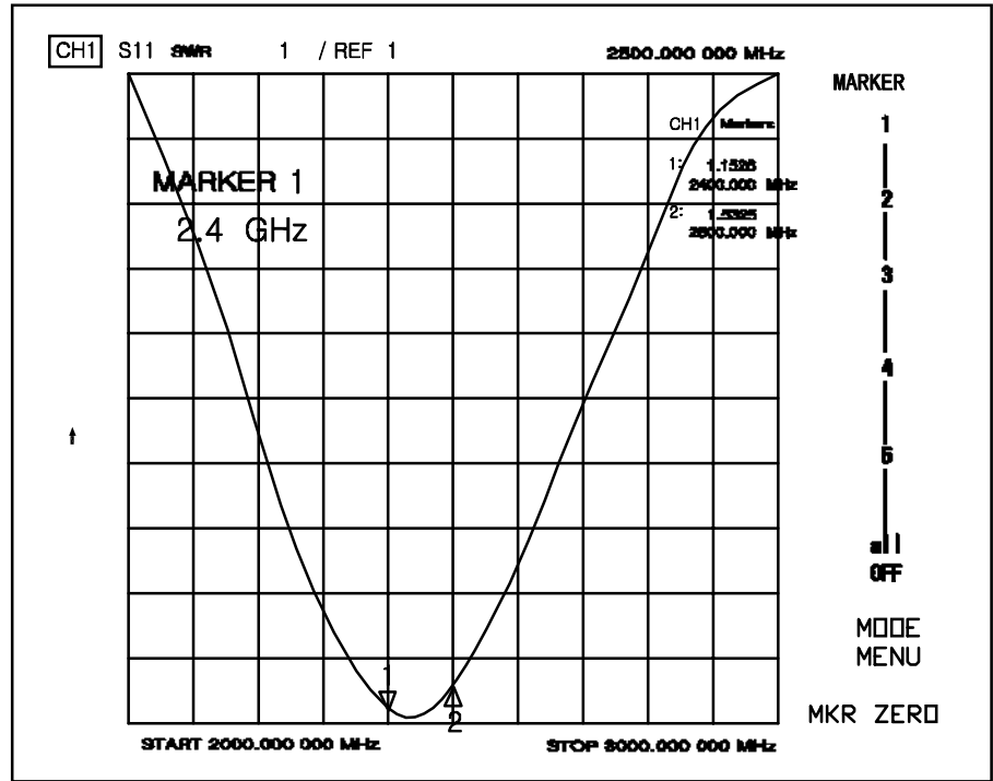
驻波图 VSWR:
