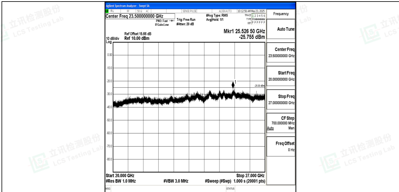
Band7_20MHz_QPSK_20850_1RB#0_20000~27000_20000~27000
