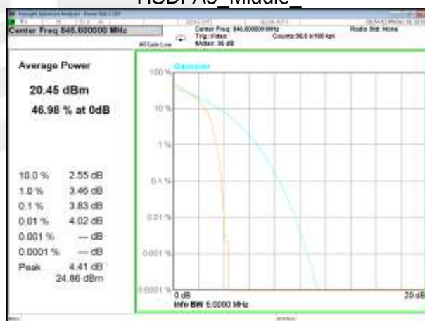
HSDPA5_Higher_
