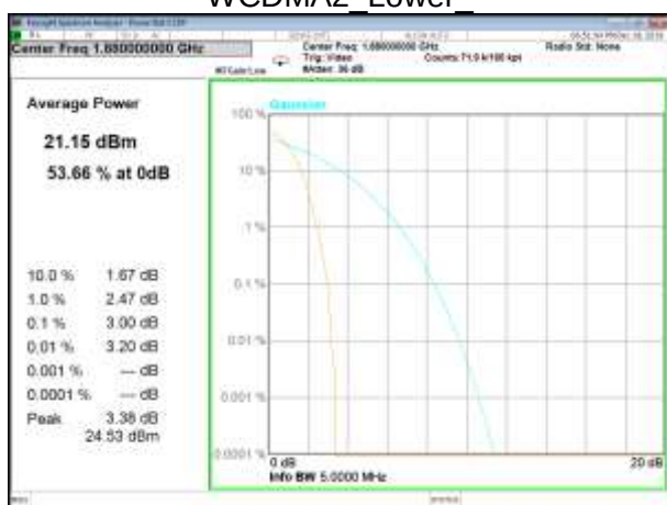
WCDMA2_Middle_
