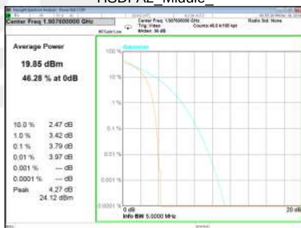
HSDPA2_Higher_
