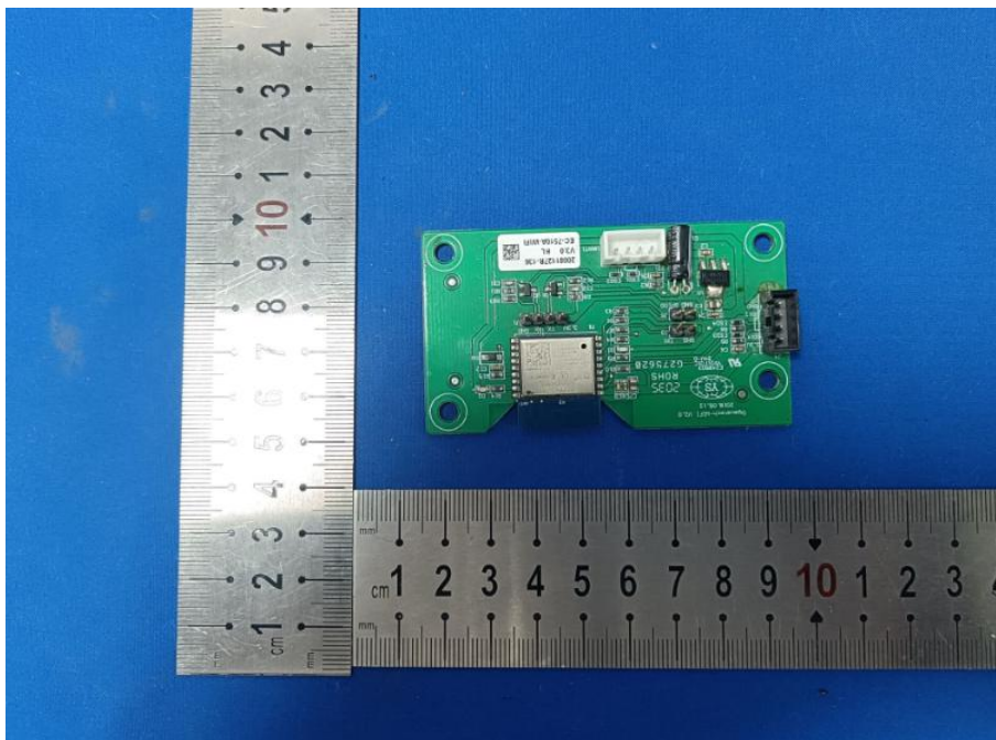
wifi module
