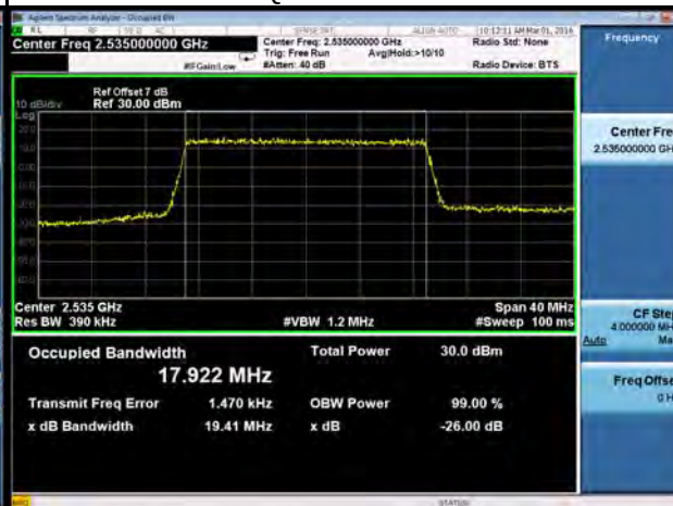
16QAM-20850
