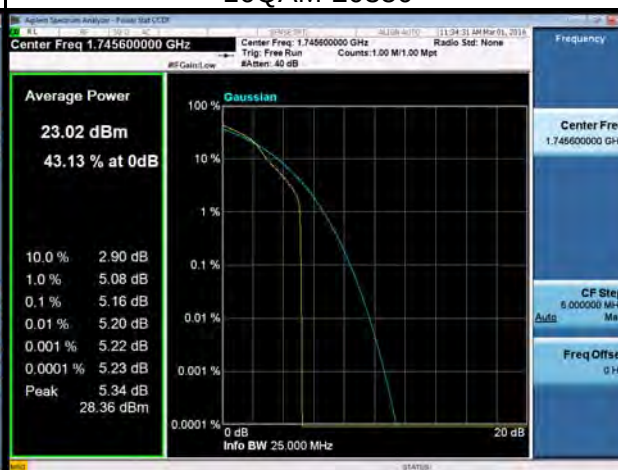
16QAM-20350
