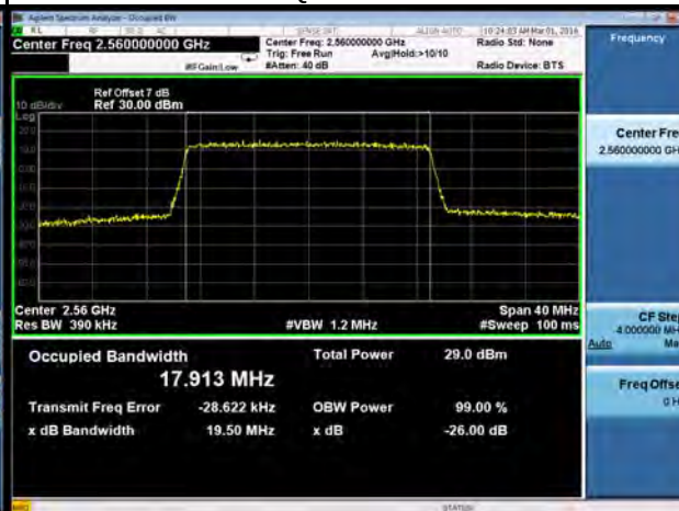
16QAM-21350
