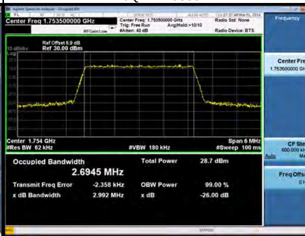
16QAM-20385
