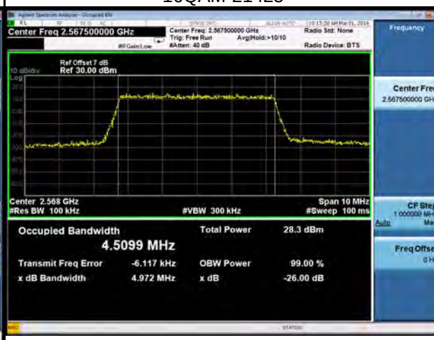
16QAM-21425
