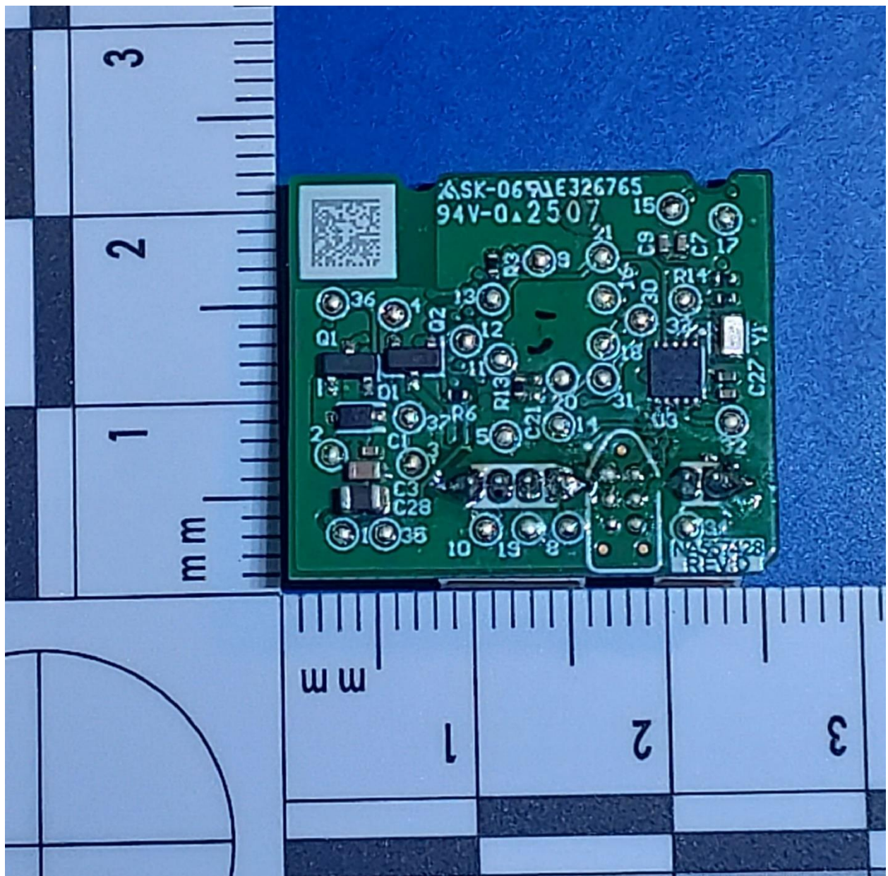
NA557427_bottom_No_Overmold
