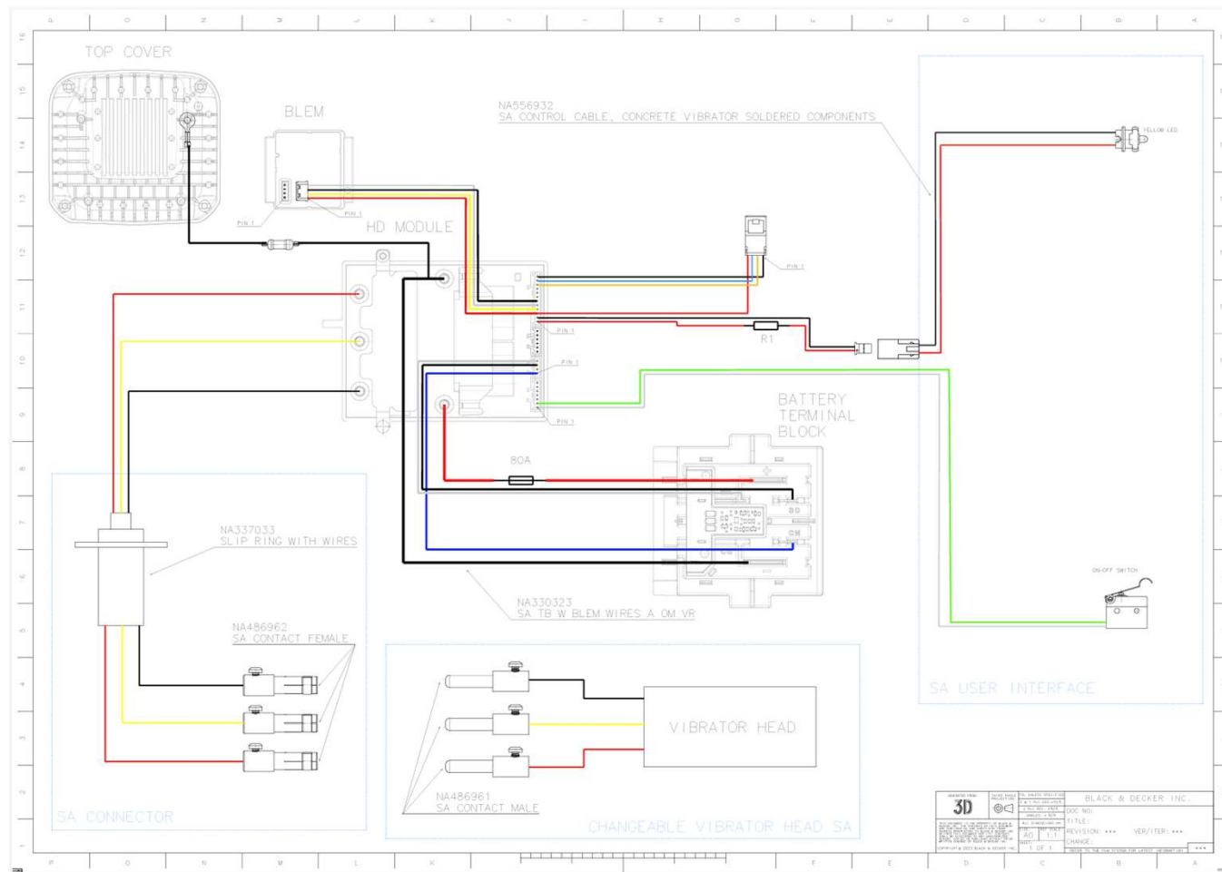
Wiring - Plan
