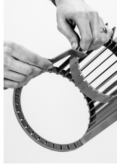
Koruyucu Muhafaza
