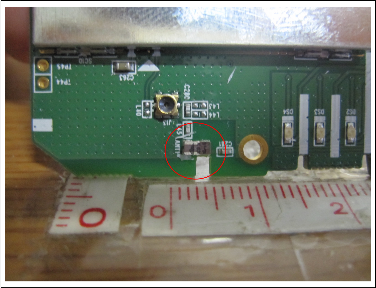
Antenna (Zigbee 1)
