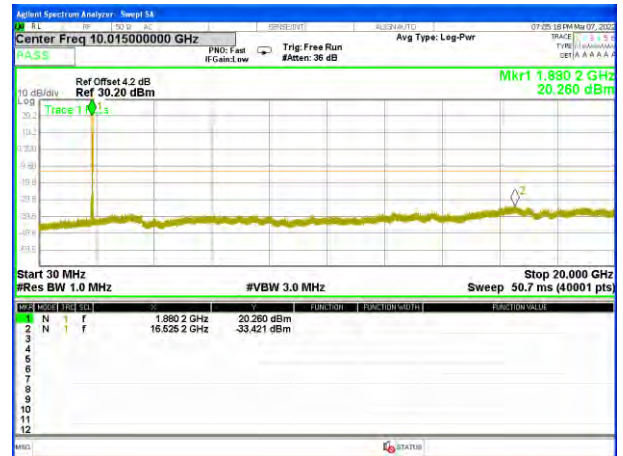
HSUPA_Band 2_Middle
