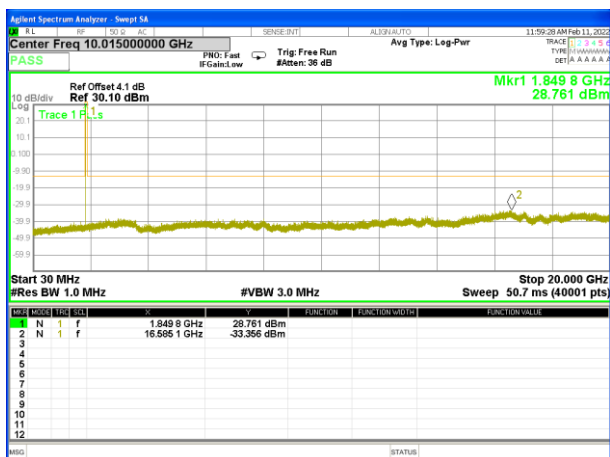
EGPRS1900_Low
