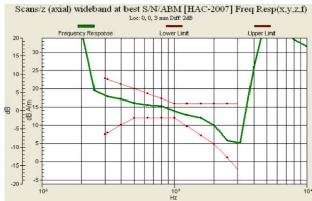
Fig. 9.1 GSM850 Ch128
