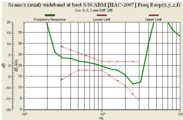
Fig. 9.3 GSM850 Ch251
