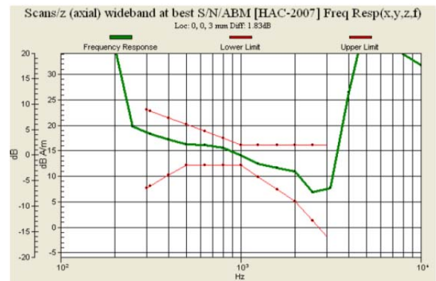
Fig. 9.2 GSM850 Ch189
