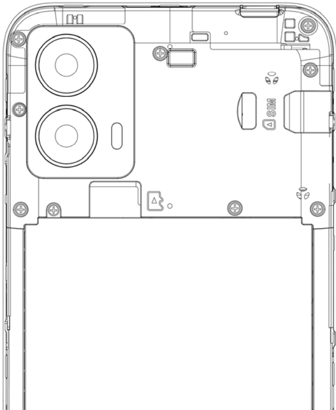
Slot para cartão SIM
