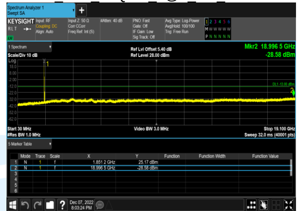
B2_20M 16QAM 1@0 CH 18900
