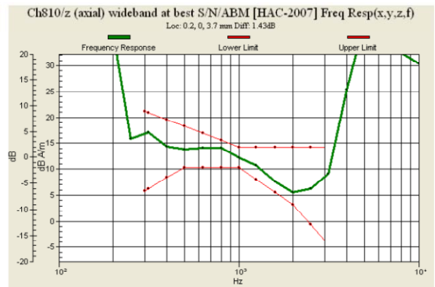
Fig. 9.6 GSM1900 Ch810
