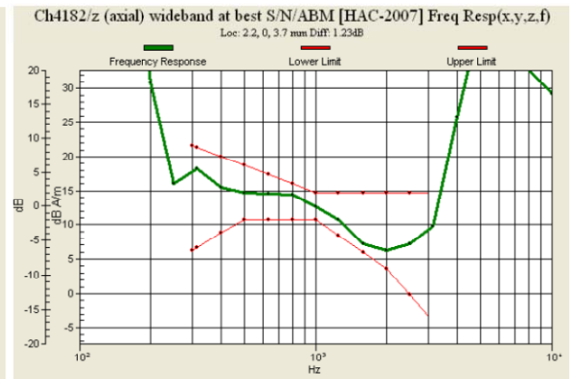
Fig. 9.2 WCDMA Band V Ch4182
