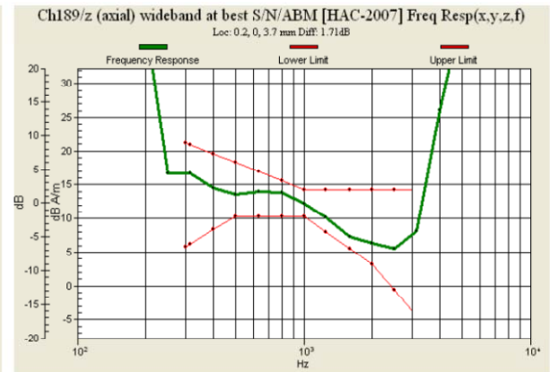
Fig. 9.2 GSM850 Ch189
