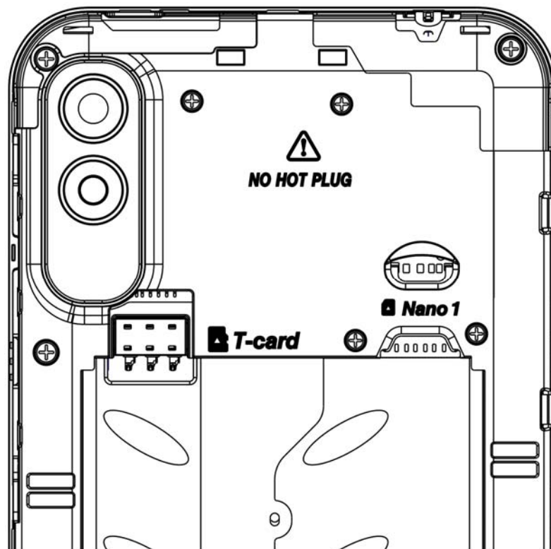
Slot para cartão SIM
