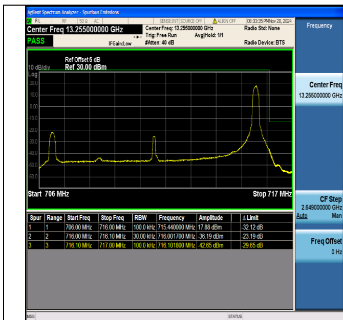
Band12 10MHz QPSK 23130 1RB#49
