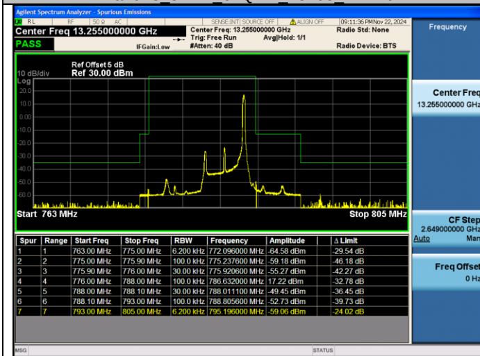
Band13 5MHz 64QAM 23255 1RB#24
