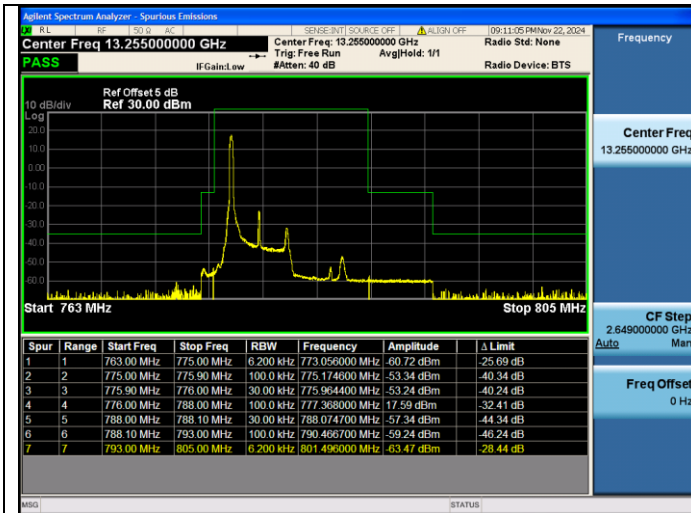
Band13 5MHz 64QAM 23205 1RB#0
