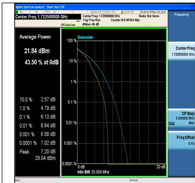
Band4-20MHz-QPSK-20175-1RB#0-PASS
