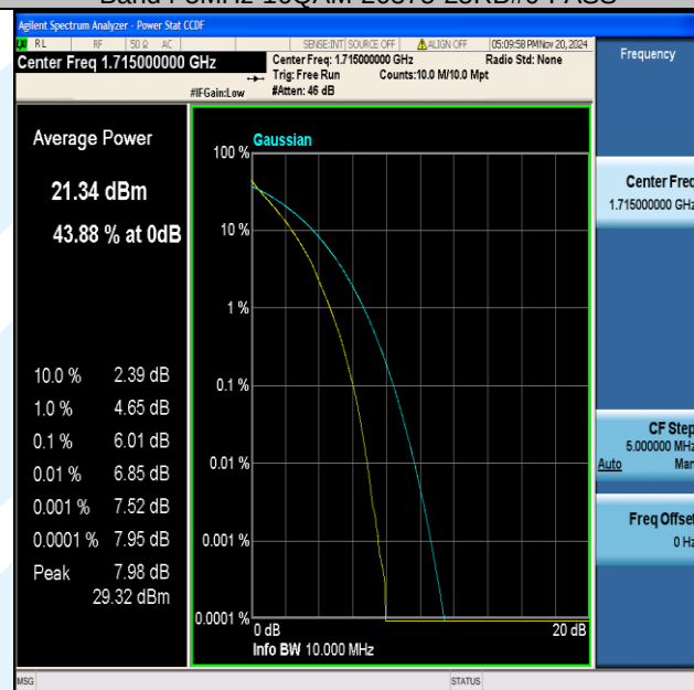
Band4-10MHz-QPSK-20000-50RB#0-PASS
