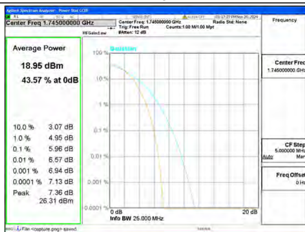
B4 / 20MHz / High CH / 64QAM
