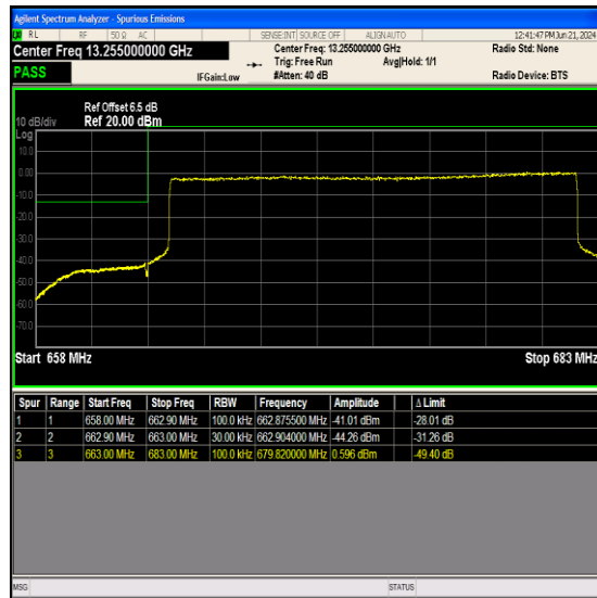
Band71_20MHz_QPSK_133222_100RB#0
