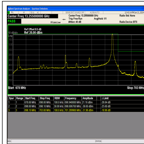
Band71_20MHz_QPSK_133372_1RB#99
