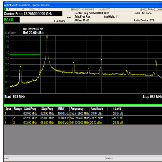
Band71_20MHz_QPSK_133222_1RB#0
