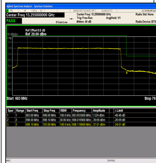
Band71_15MHz_QPSK_133397_75RB#0
