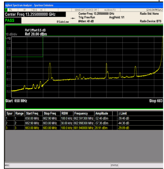
Band71_20MHz_QPSK_133222_1RB#99
