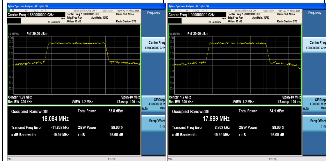
Band2-20MHz-QPSK-18900-100RB#0-PASS
