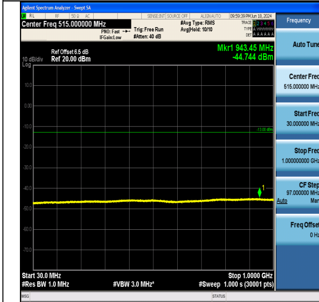
EGPRS1900-810-2-30~1000MHz-PASS
