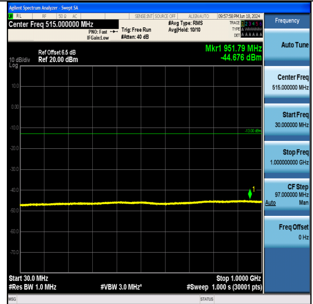
EGPRS1900-661-2-30~1000MHz-PASS
