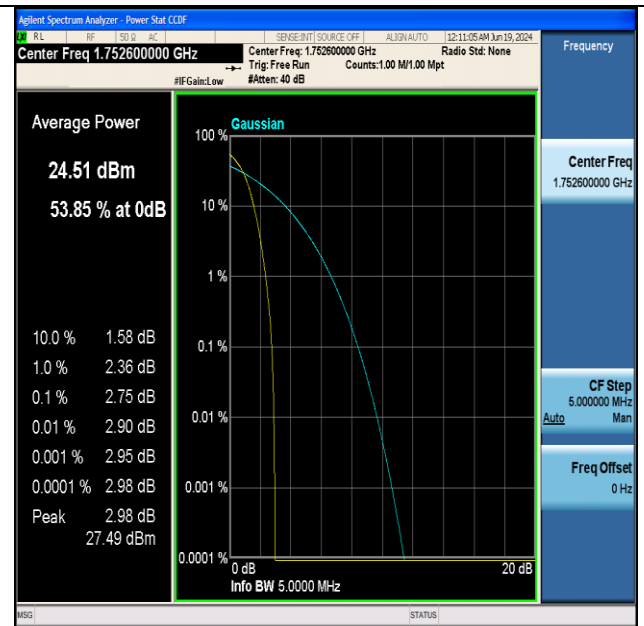
Band4-1513-PASS
