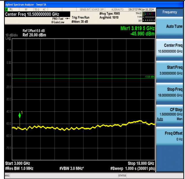
GPRS1900-810-0-3000~18000MHz-PASS
