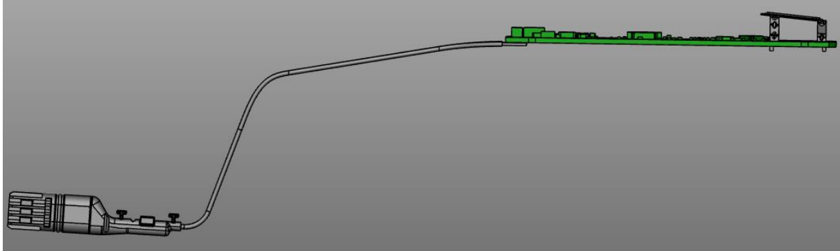
Figure 1: PCBA BMW Mini Side view
