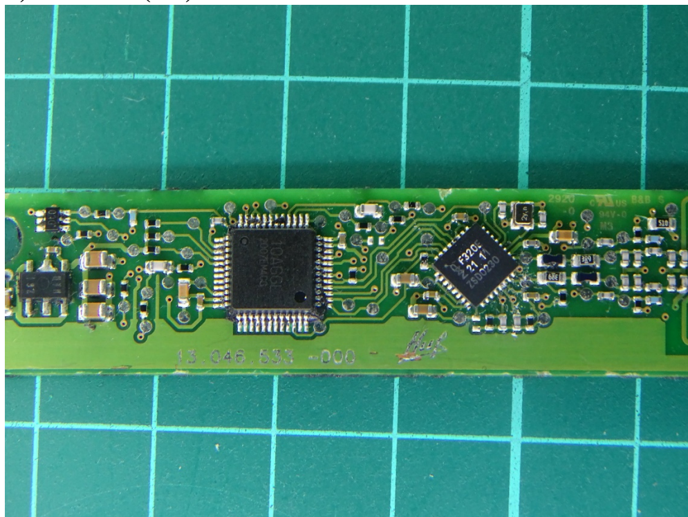
(17) EUT Photo (G26)
