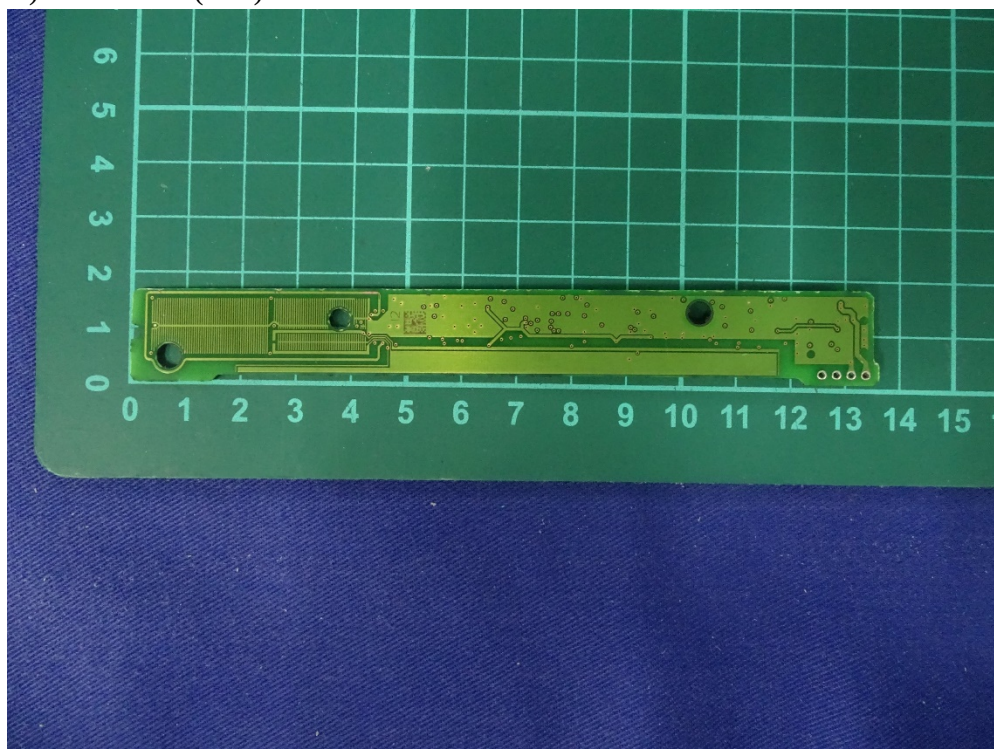
(14) EUT Photo (G26)
