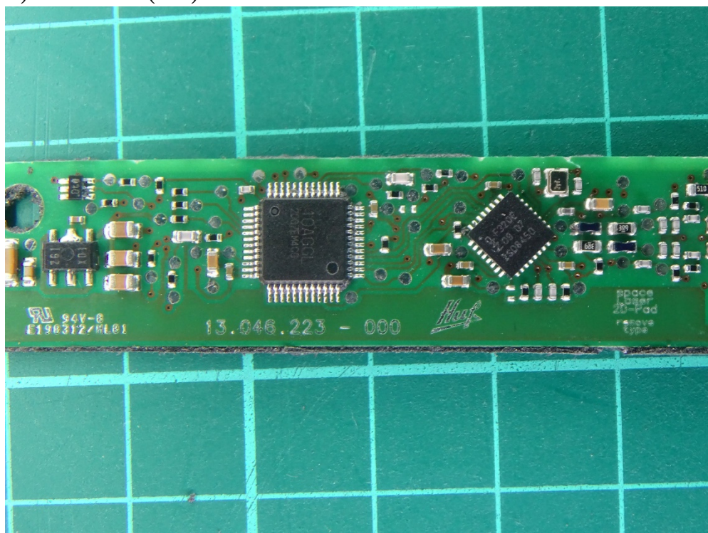
(22) EUT Photo (U06)
