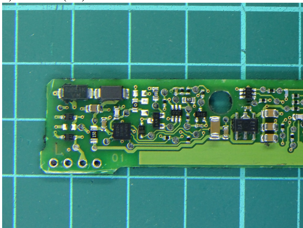
(16) EUT Photo (G26)
