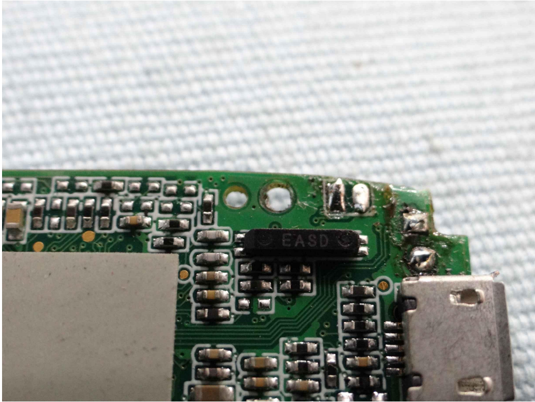
Y2 Crystal
