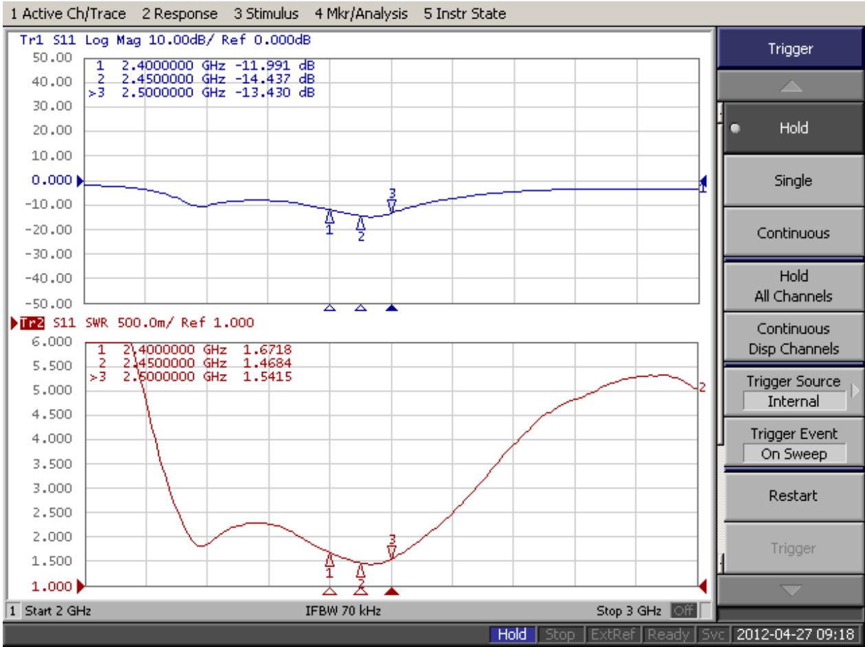
天线返回损失和电压驻波比对应波形图
