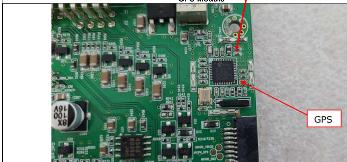
GPS Module
