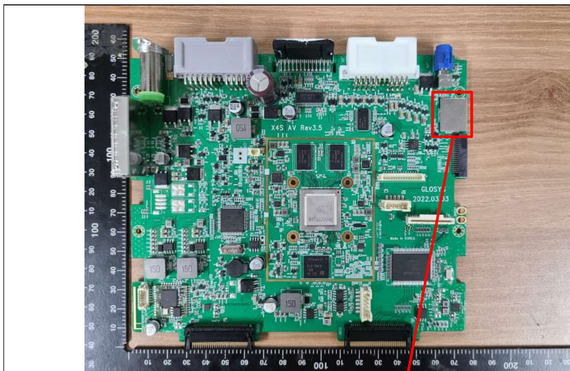
GPS Module
