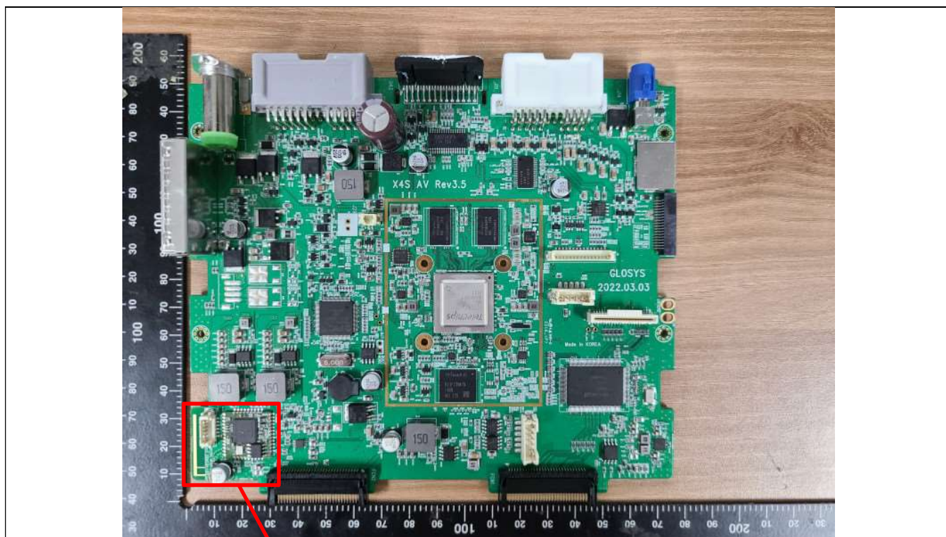
Bluetooth Module & Antenna
