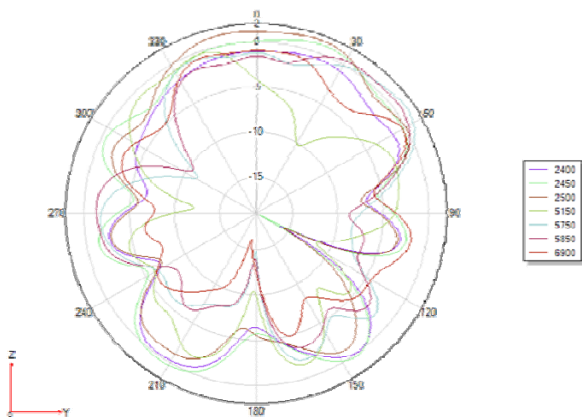
Phi 90°
