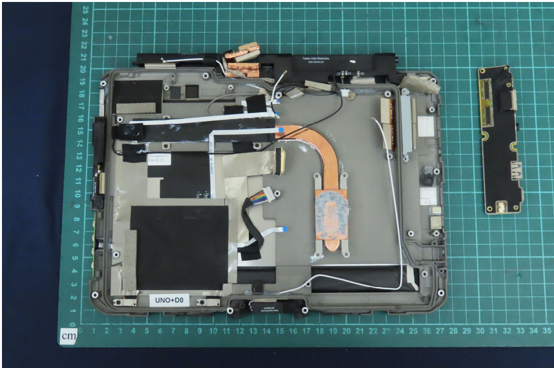
(37) EUT Photo
