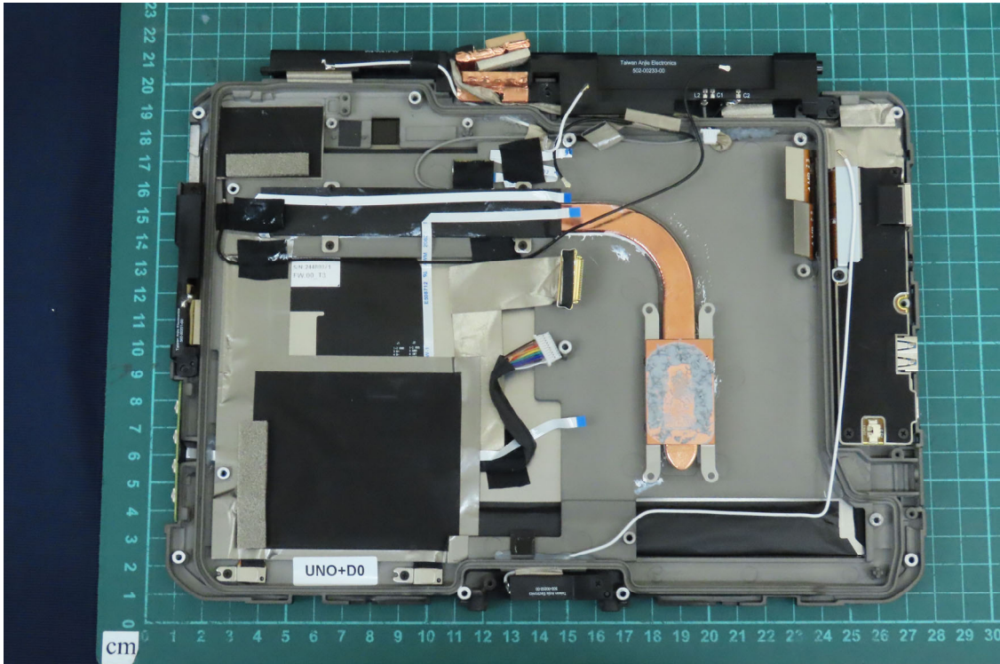
(36) EUT Photo
