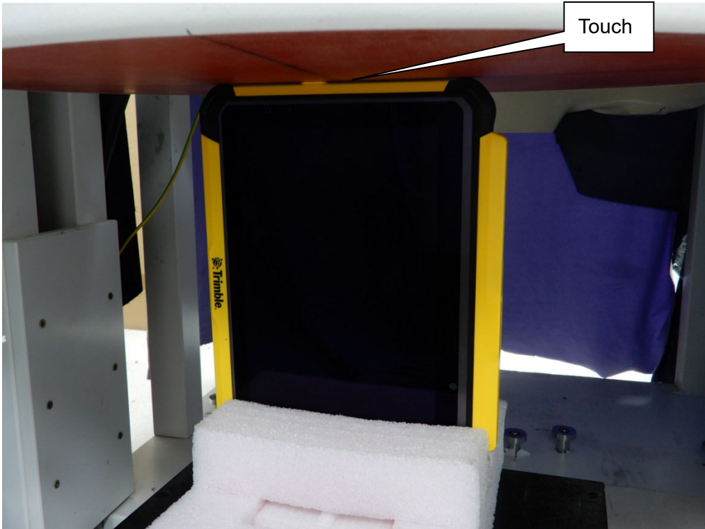
EUT Left-side_0mm
