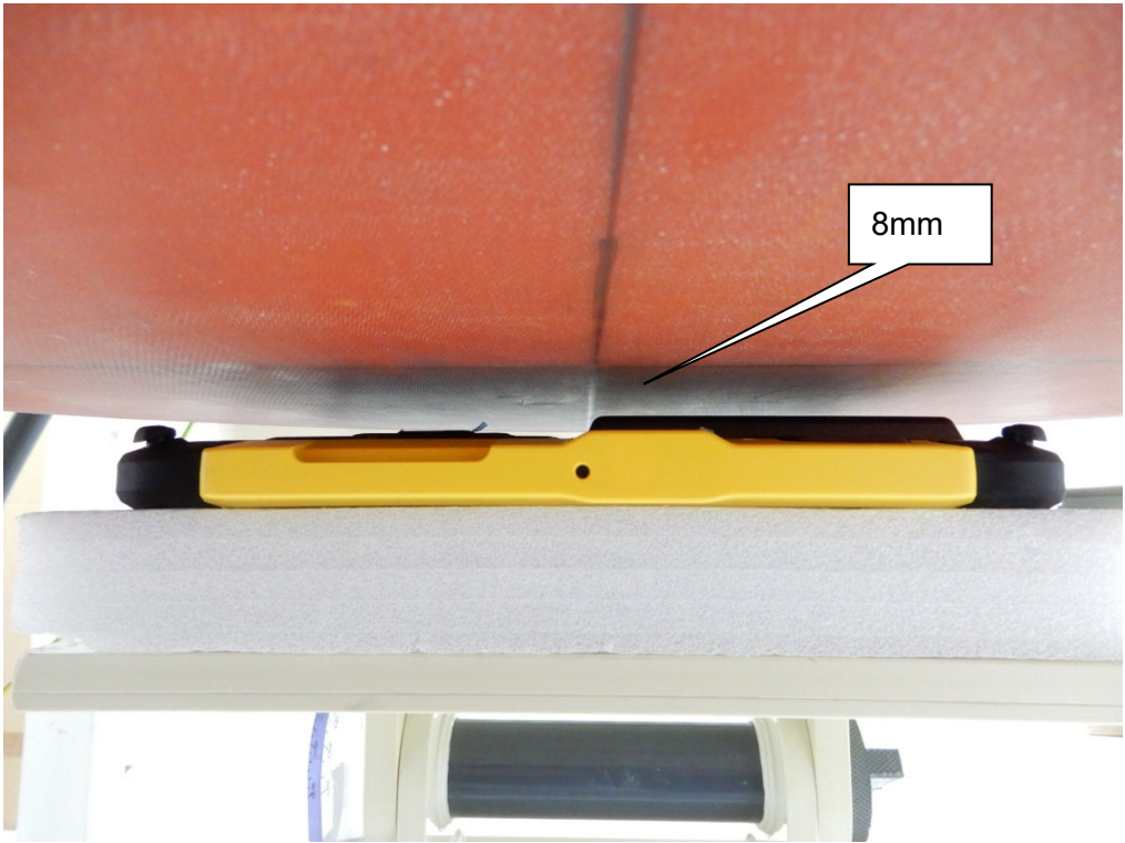
EUT Back_8mm
