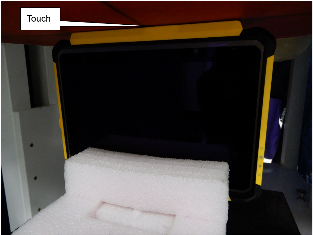
EUT Top_0mm
