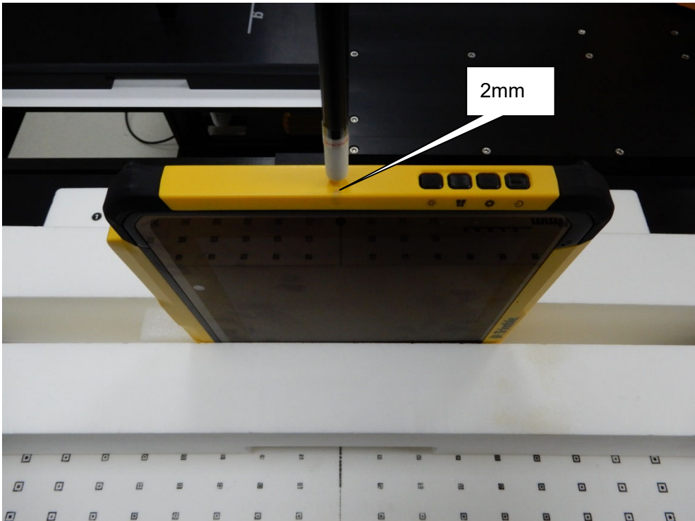
EUT Right-side_PD_2mm
