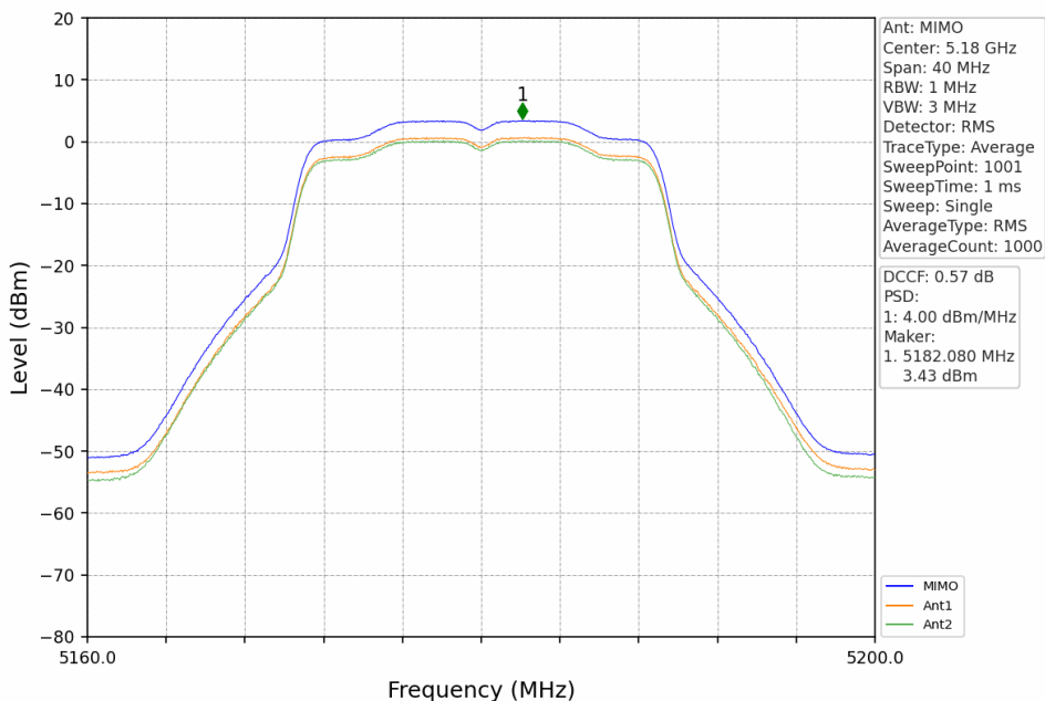
802.11n(HT20)_LCH_5180MHz_MIMO_NTNV
