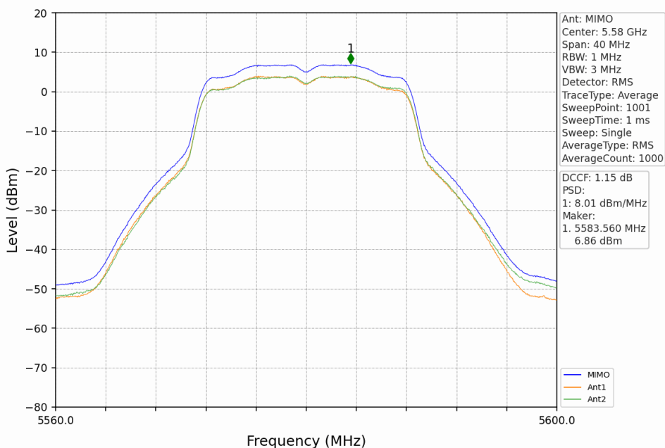
802.11a_MCH_5580MHz_MIMO_NTNV
