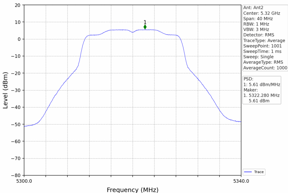
802.11n(HT20)_HCH_5320MHz_Ant2_NTNV
