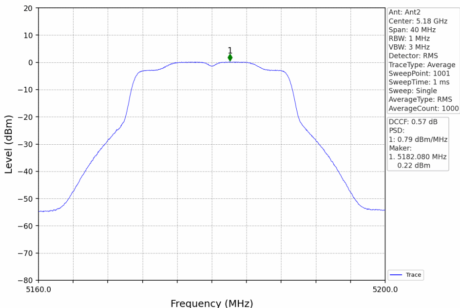
802.11n(HT20)_LCH_5180MHz_MIMO_NTNV
