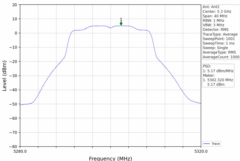
802.11n(HT20)_MCH_5300MHz_MIMO_NTNV
