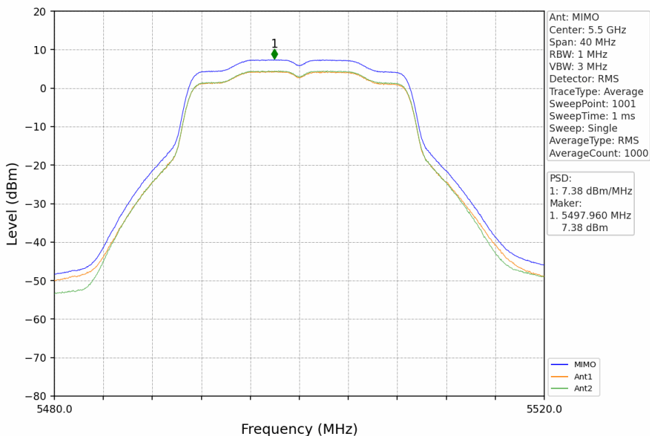
802.11n(HT20)_LCH_5500MHz_MIMO_NTNV
