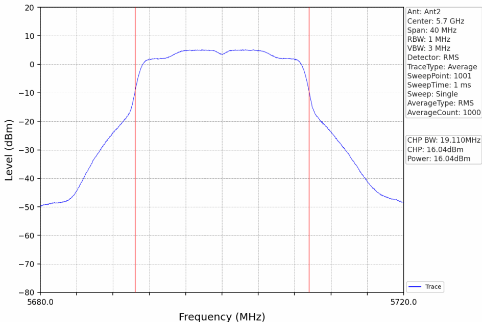
802.11n(HT20)_HCH_5700MHz_Ant2_NTNV
