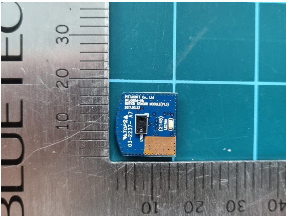
<PCB 3 - Rear>
