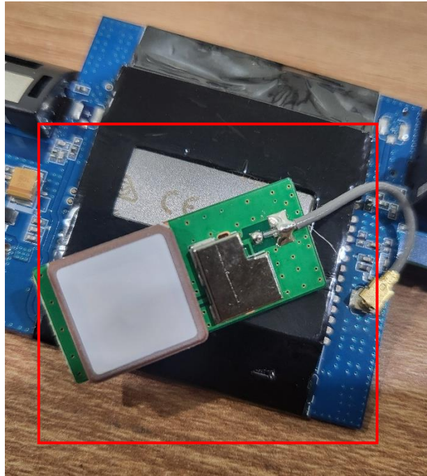
GPS Antenna
