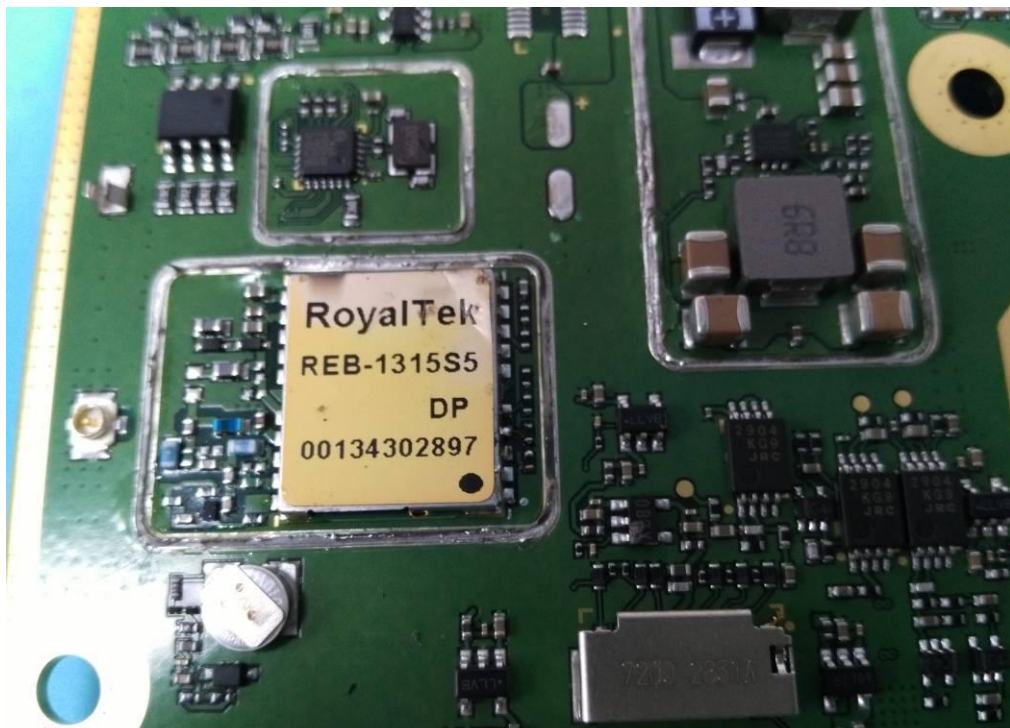
GPS module
