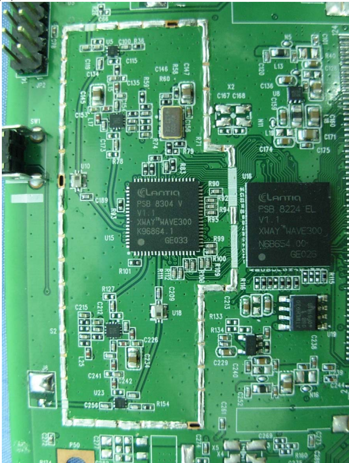
(14) EUT Photo
