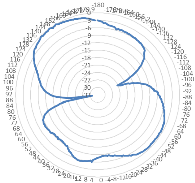
Diagramme de rayonnement Normalisée, dB
