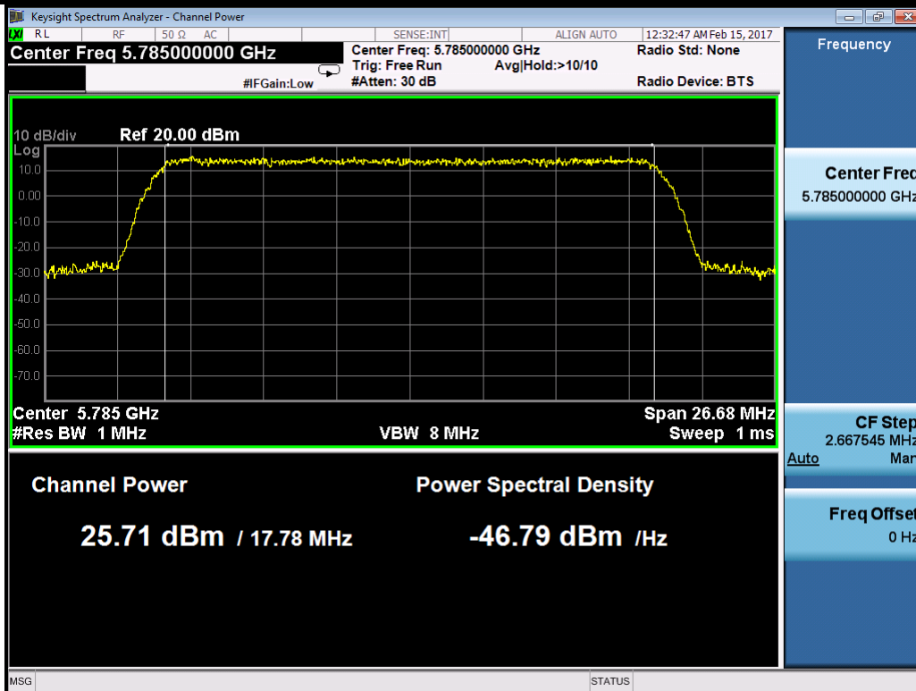
64QAM-5785MHz
