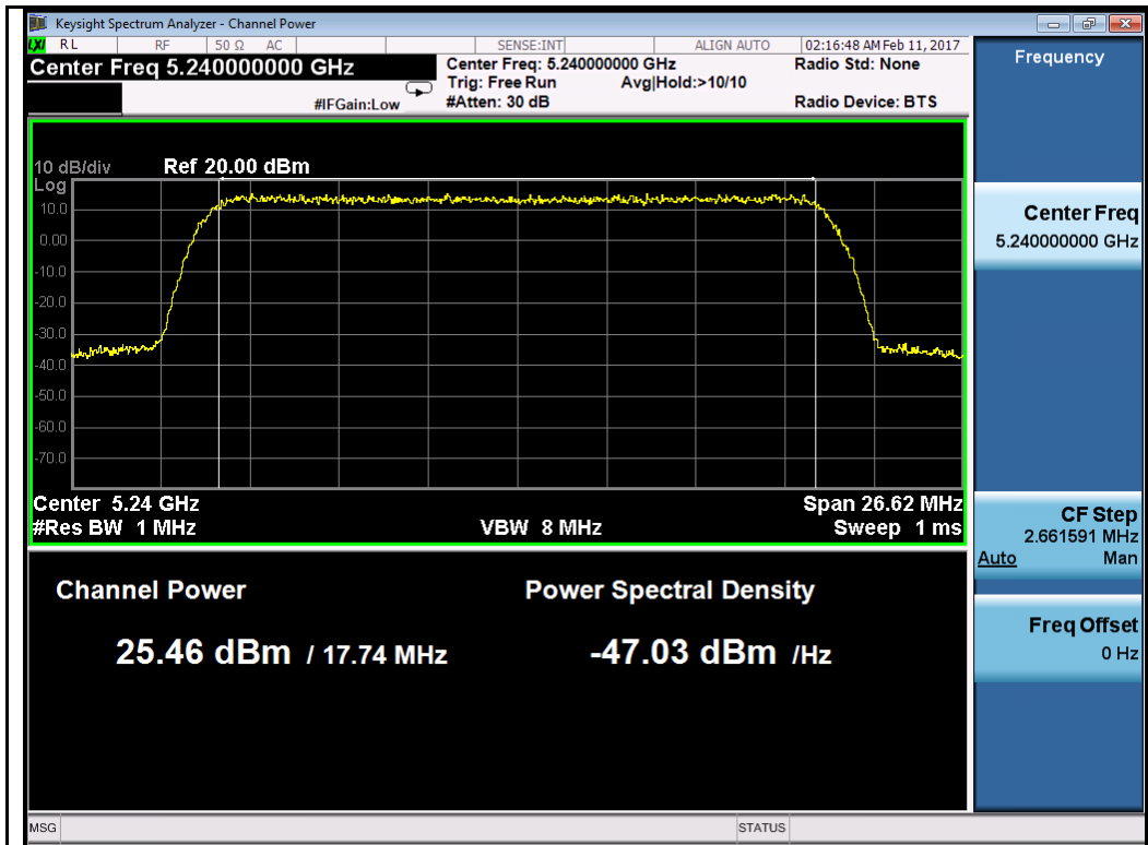
QPSK-5240MHz
