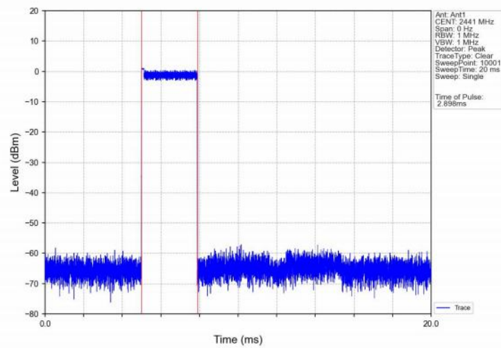
8DPSK_3DH5_HOPP_Ant1_NTNV
