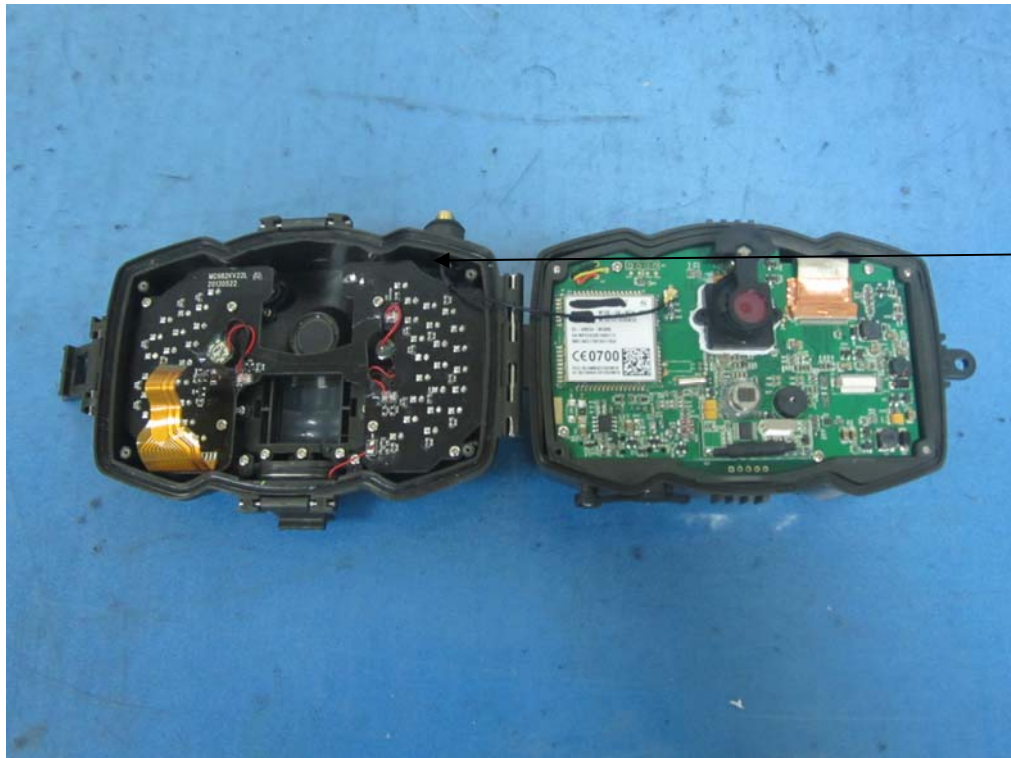
GSM Antenna
