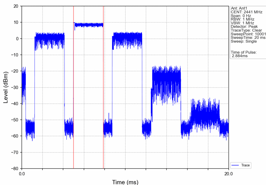
8DPSK_3DH5_HOPP_Ant1_NTNV
