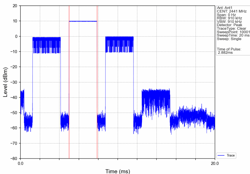
GFSK_DH5_HOPP_Ant1_NTNV
