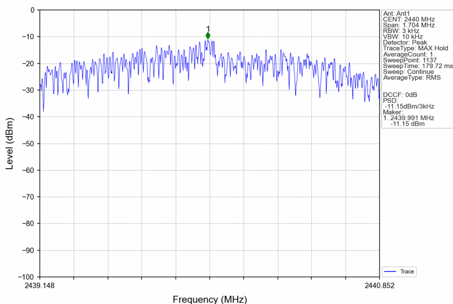
2M_MCH_2440MHz_Ant1_NTNV
