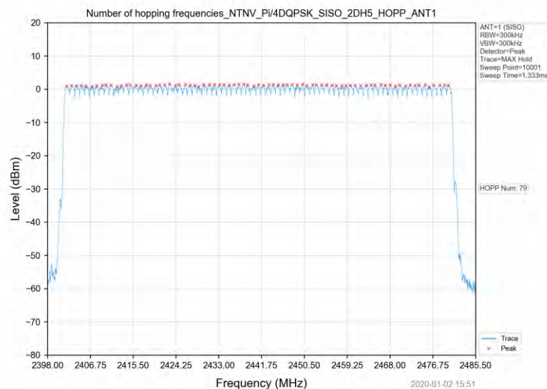
Pi/4DQPSK_Hopping_2DH5_SISO_ANT1
