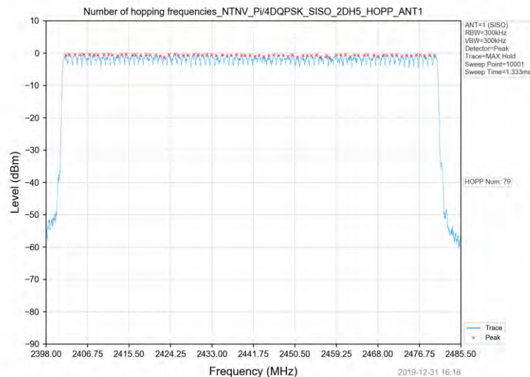
Pi/4DQPSK_Hopping_2DH5_SISO_ANT1
