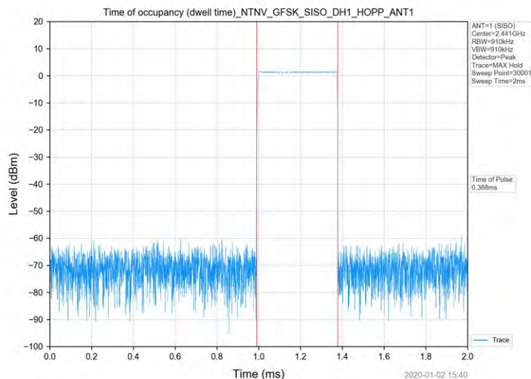
GFSK_Hopping_DH1_SISO_ANT1
