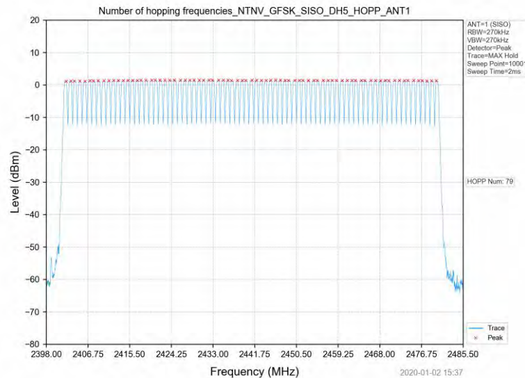
GFSK_Hopping_DH5_SISO_ANT1
