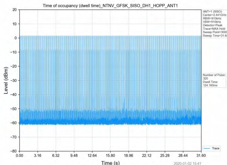
GFSK_Hopping_DH1_SISO_ANT1
