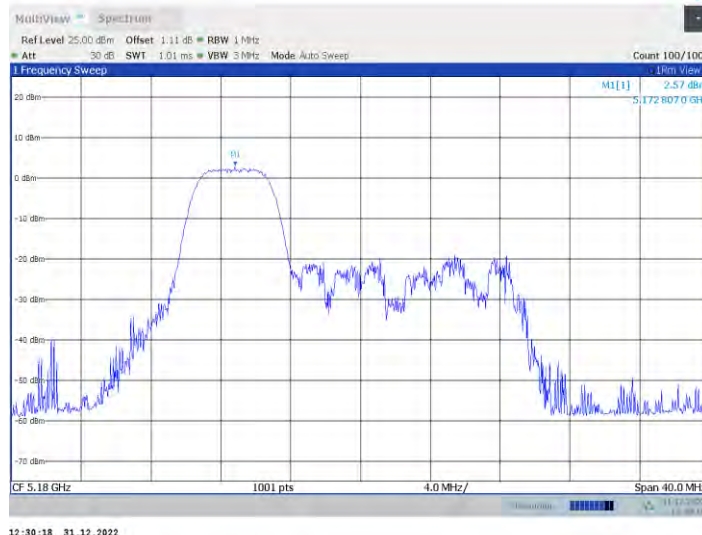
11ax20MIMO Ant1 5180 52Tone_RU37
