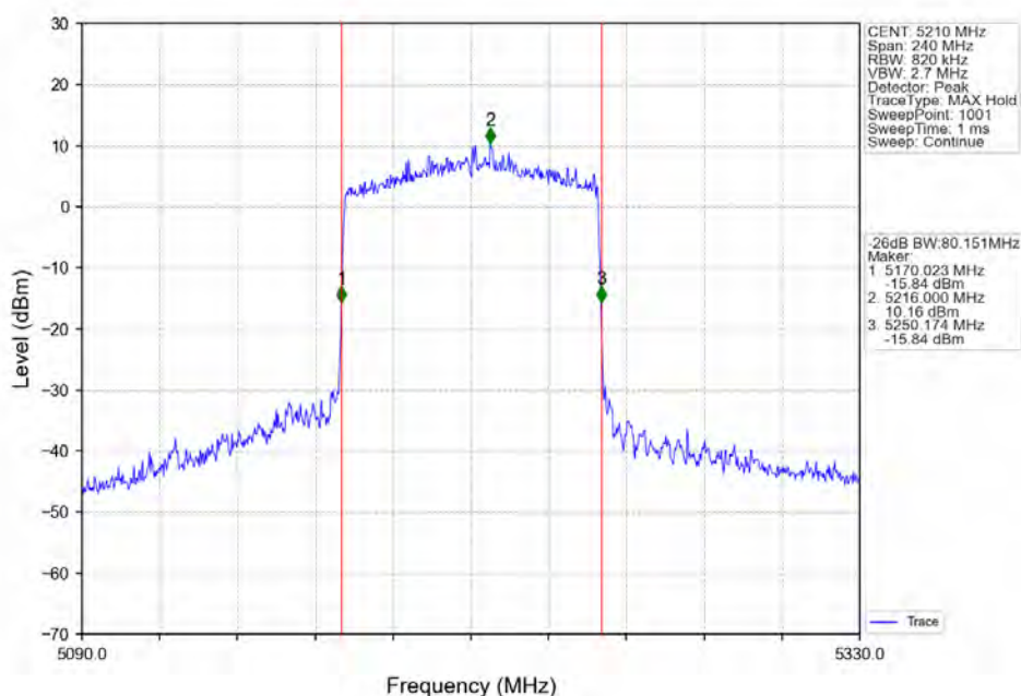
802.11ax(HE80)_MCH_5210MHz_RU996_Left_Ant1_NTNV
