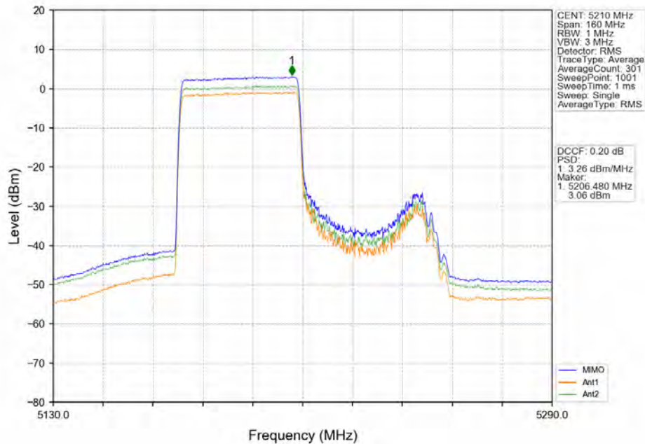
802.11ax(HE80)_MCH_5210MHz_RU484_Left_MIMO_NTNV
