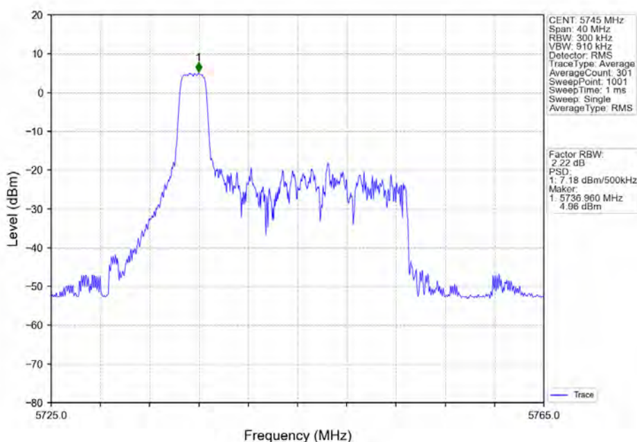
802.11ax(HE20)_LCH_5745MHz_RU26_Left_Ant1_NTNV
