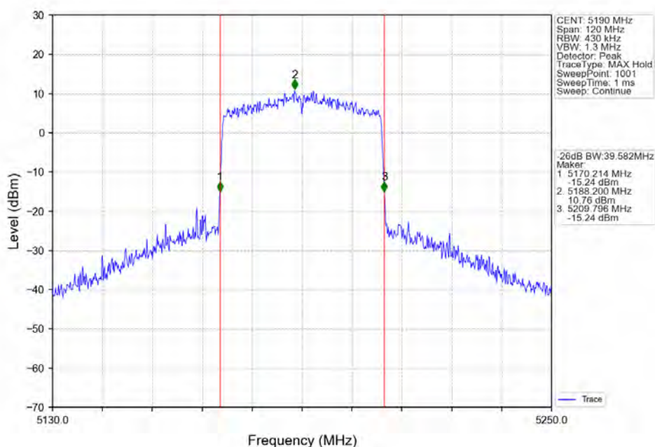
802.11ax(HE40)_LCH_5190MHz_RU484_Left_Ant1_NTNV
