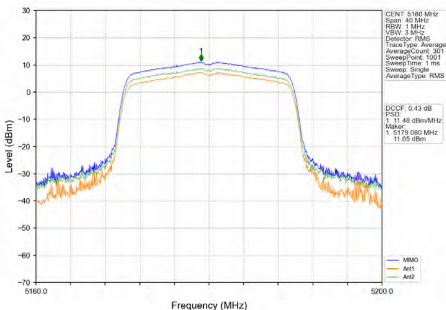
802.11ax(HE20)_LCH_5180MHz_RU242_Left_MIMO_NTNV
