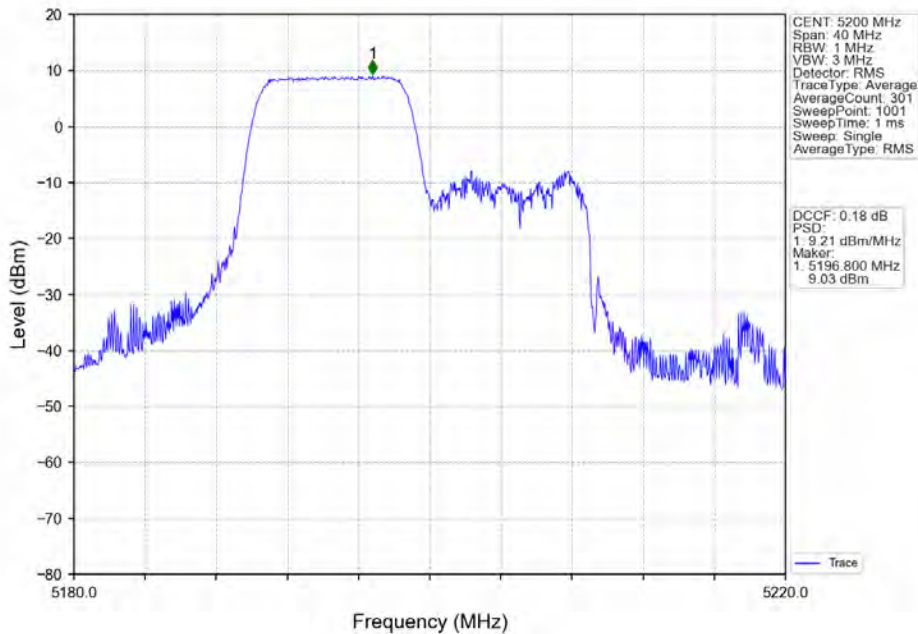
802.11ax(HE20)_MCH_5200MHz_RU106_Left_Ant2_NTNV
