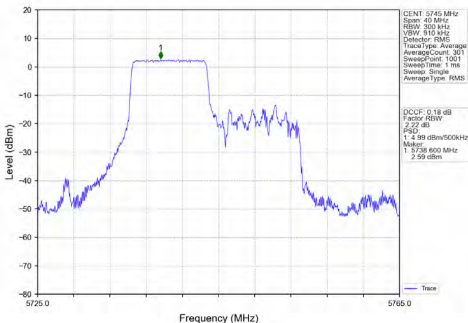
802.11ax(HE20)_LCH_5745MHz_RU106_Left_Ant2_NTNV
