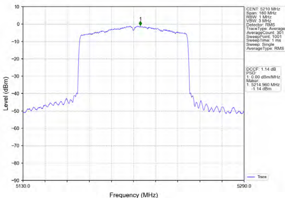
802.11ax(HE80)_MCH_5210MHz_RU996_Left_Ant1_NTNV
