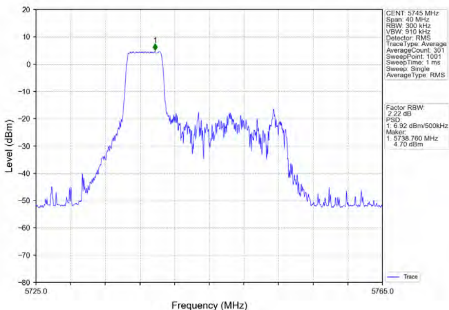
802.11ax(HE20)_LCH_5745MHz_RU52_Left_Ant1_NTNV
