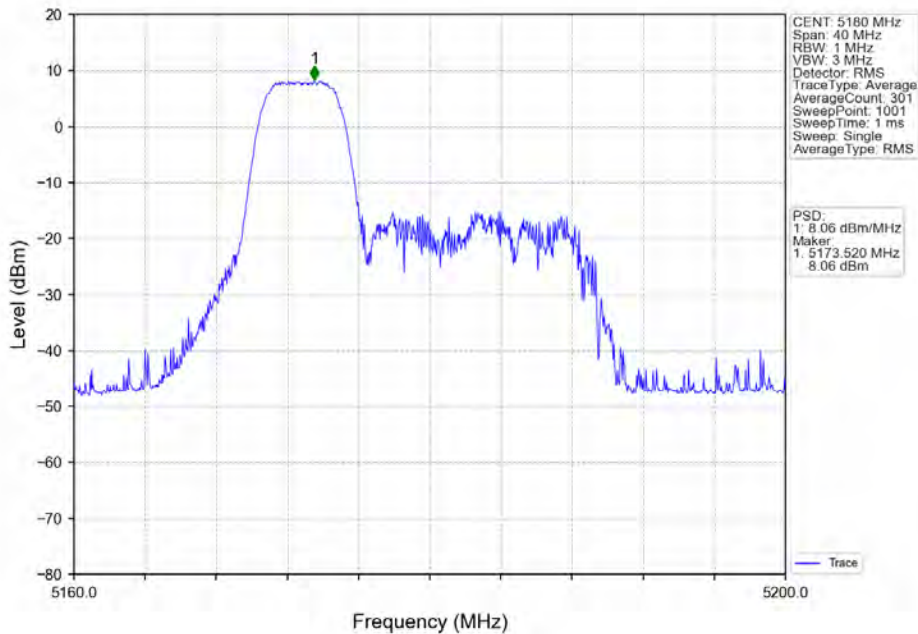
802.11ax(HE20)_LCH_5180MHz_RU52_Left_Ant2_NTNV
