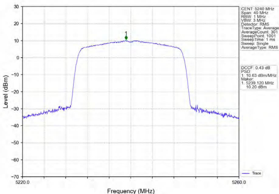
802.11ax(HE20)_HCH_5240MHz_RU242_Left_Ant2_NTNV
