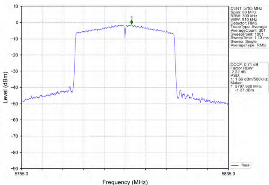
802.11ax(HE40)_HCH_5795MHz_RU484_Left_Ant1_NTNV
