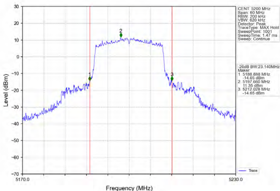
802.11ax(HE20)_MCH_5200MHz_RU242_Left_Ant2_NTNV
