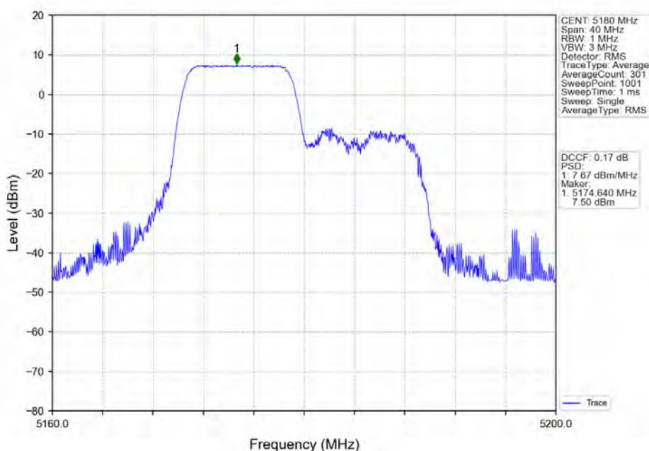
802.11ax(HE20)_LCH_5180MHz_RU106_Left_Ant1_NTNV
