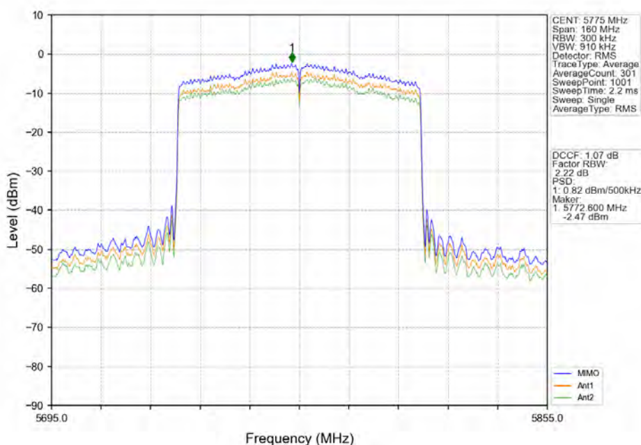
802.11ax(HE80)_MCH_5775MHz_RU996_Left_MIMO_NTNV
