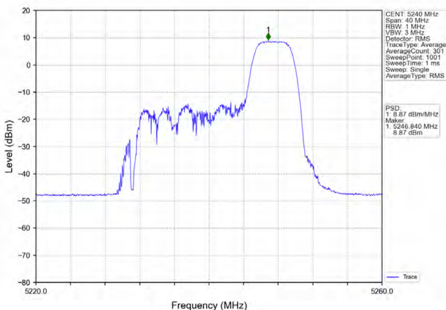
802.11ax(HE20)_HCH_5240MHz_RU52_Right_Ant1_NTNV
