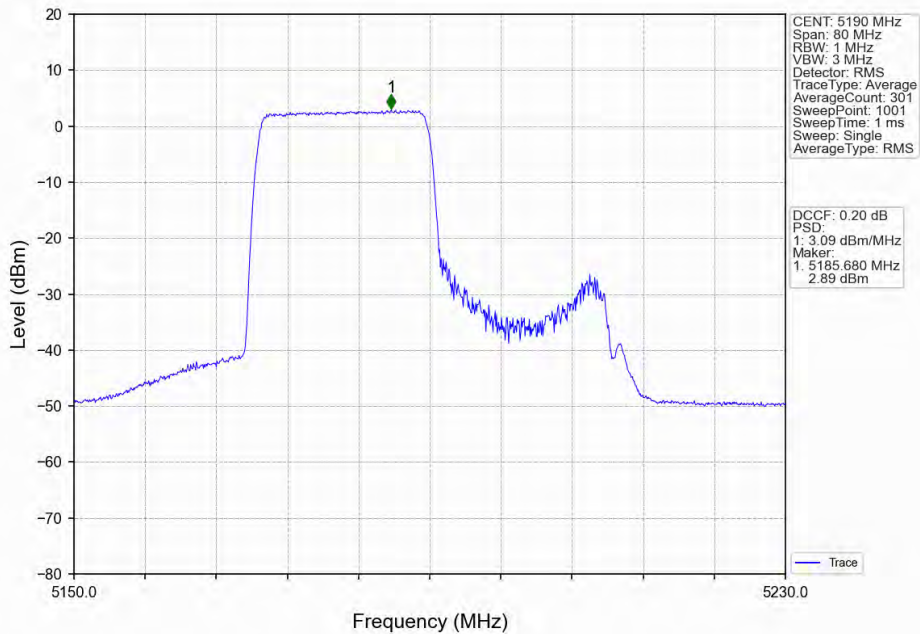
802.11ax(HE40)_LCH_5190MHz_RU242_Left_Ant1_NTNV
