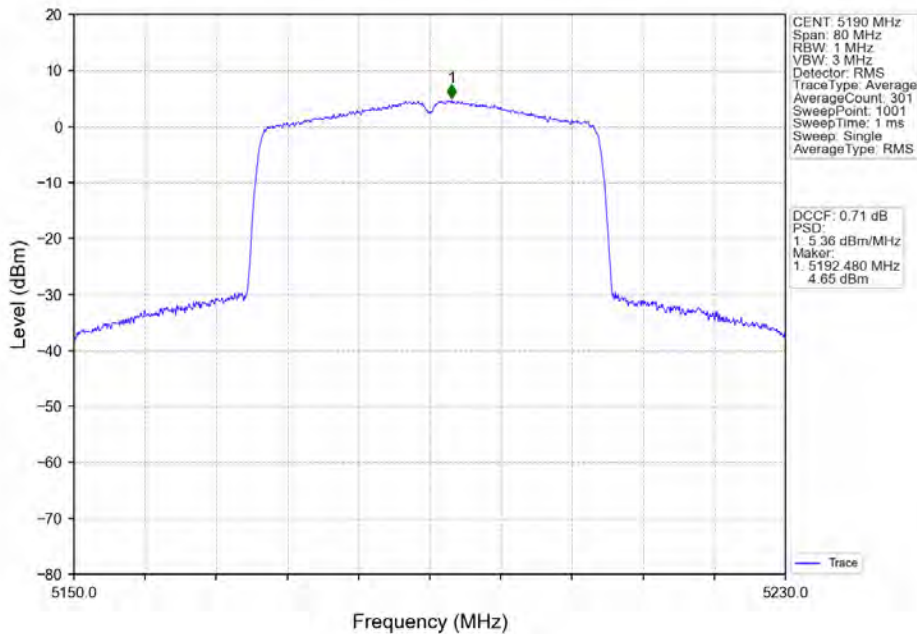
802.11ax(HE40)_LCH_5190MHz_RU484_Left_Ant2_NTNV
