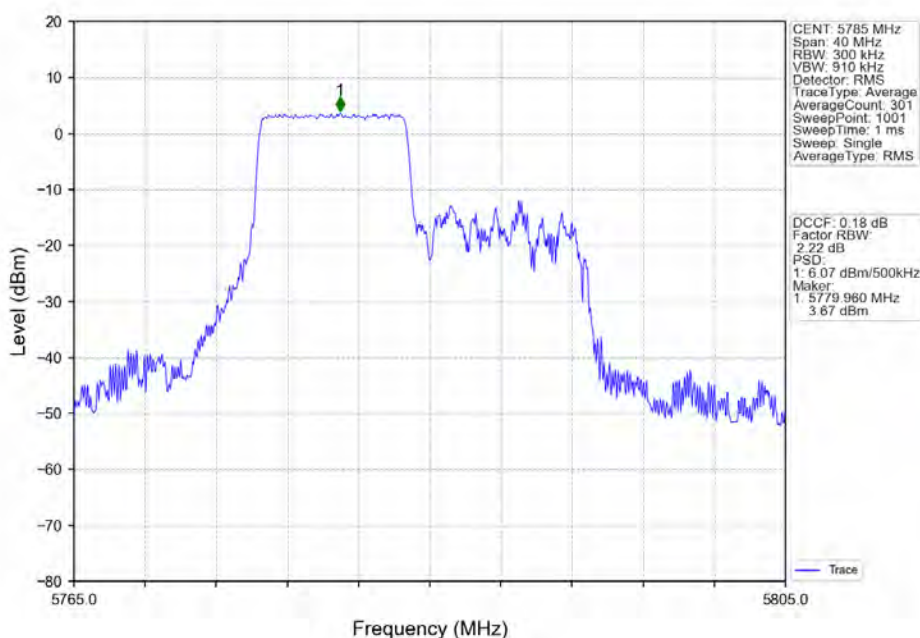
802.11ax(HE20)_MCH_5785MHz_RU106_Left_Ant1_NTNV
