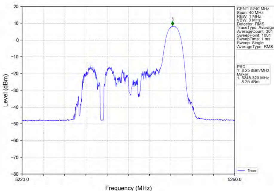
802.11ax(HE20)_HCH_5240MHz_RU26_Right_Ant1_NTNV
