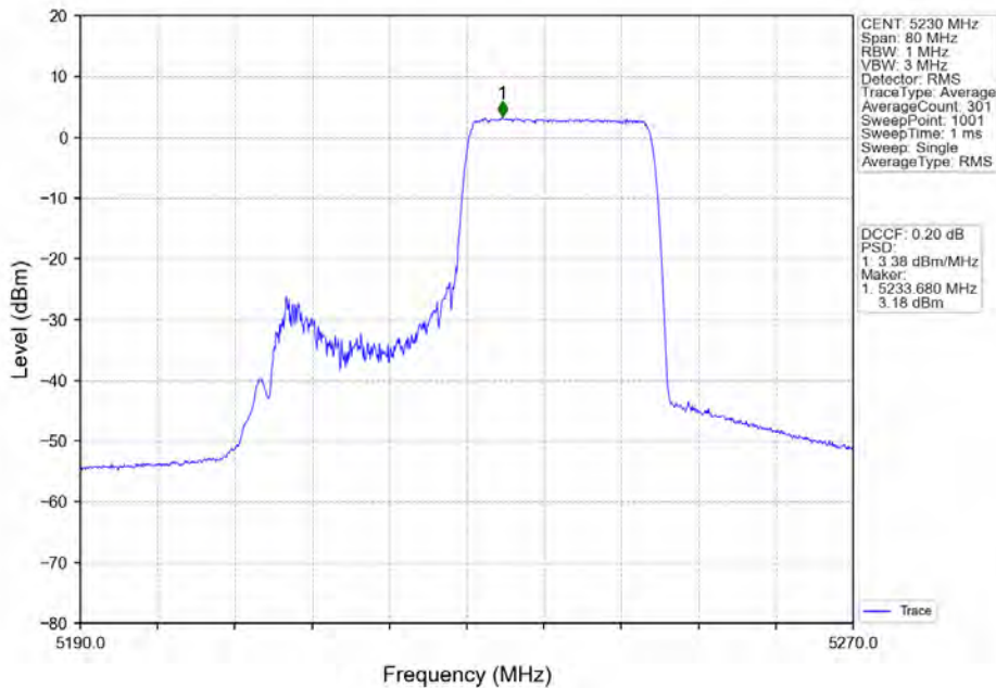
802.11ax(HE40)_HCH_5230MHz_RU242_Right_Ant1_NTNV
