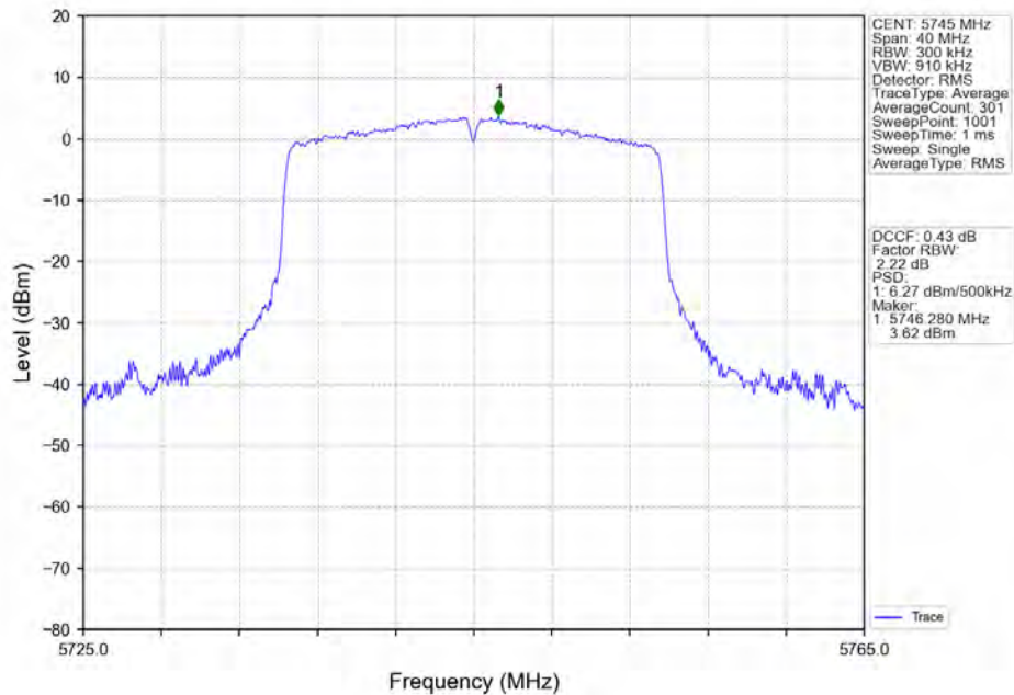
802.11ax(HE20)_LCH_5745MHz_RU242_Left_Ant2_NTNV
