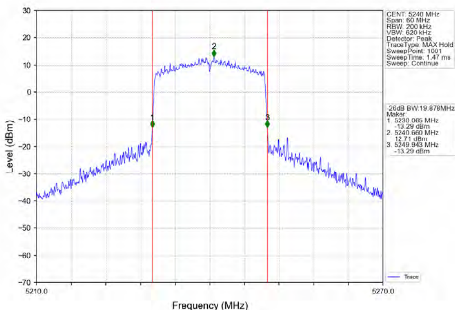
802.11ax(HE20)_HCH_5240MHz_RU242_Left_Ant2_NTNV
