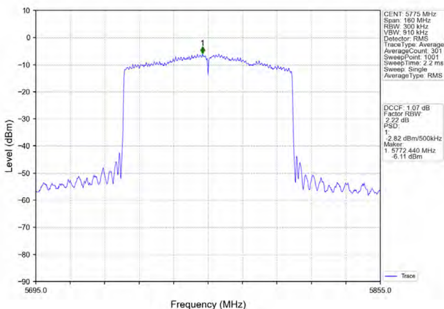
802.11ax(HE80)_MCH_5775MHz_RU996_Left_Ant2_NTNV
