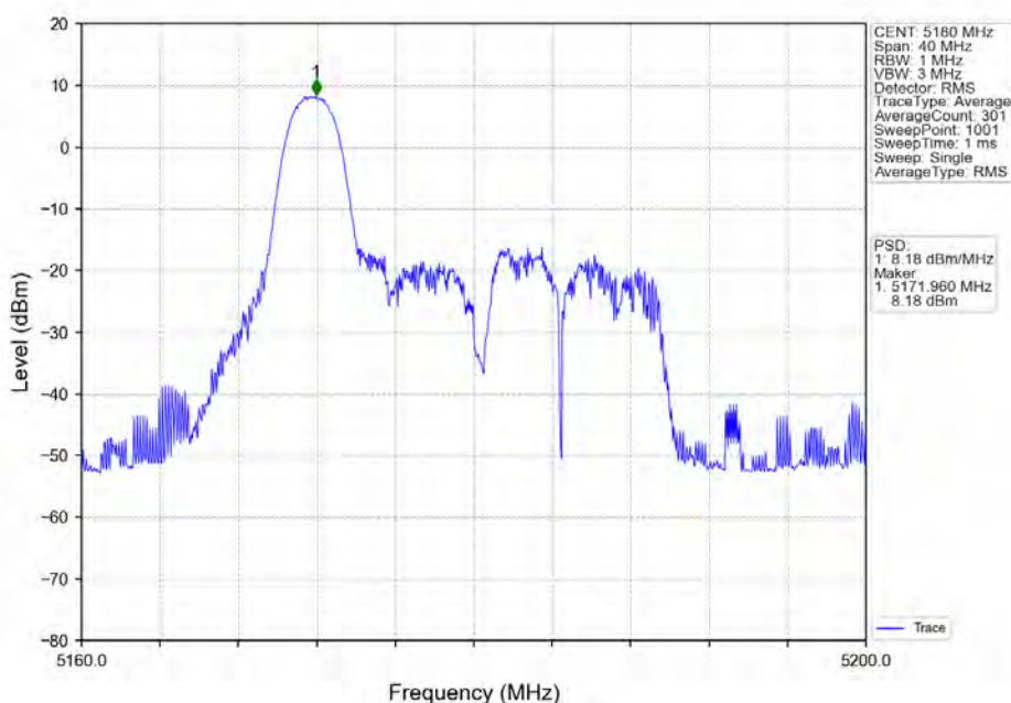
802.11ax(HE20)_LCH_5180MHz_RU26_Left_Ant2_NTNV
