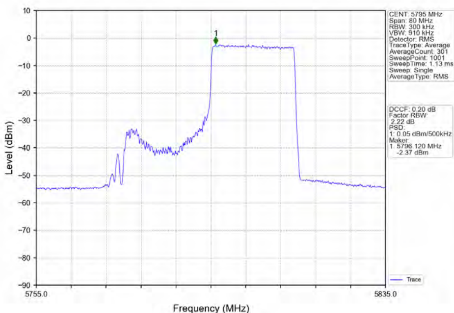
802.11ax(HE40)_HCH_5795MHz_RU242_Right_Ant2_NTNV
