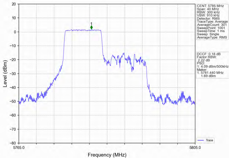
802.11ax(HE20)_MCH_5785MHz_RU106_Left_Ant2_NTNV
