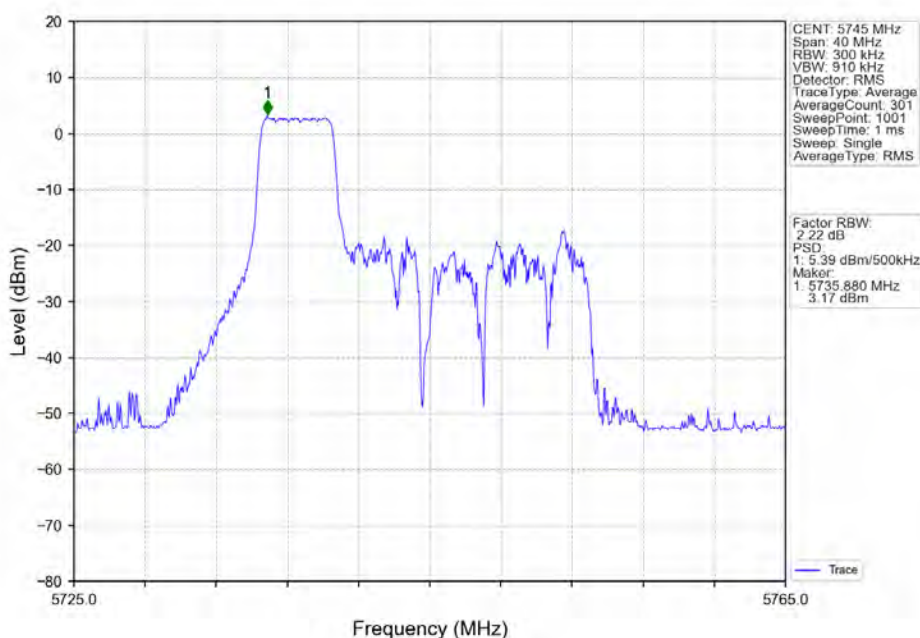
802.11ax(HE20)_LCH_5745MHz_RU52_Left_Ant2_NTNV
