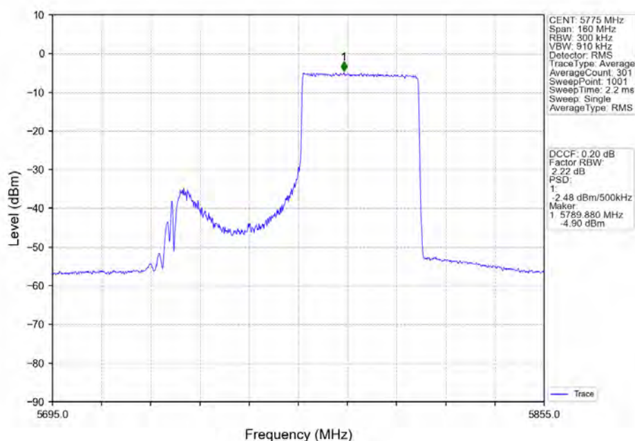
802.11ax(HE80)_MCH_5775MHz_RU484_Right_Ant1_NTNV
