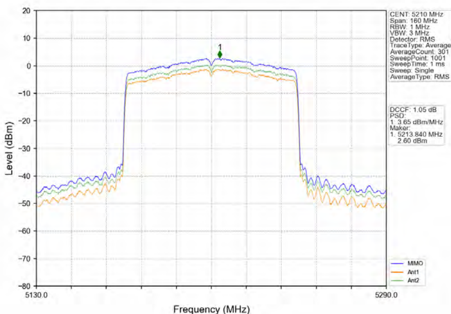
802.11ax(HE80)_MCH_5210MHz_RU996_Left_MIMO_NTNV
