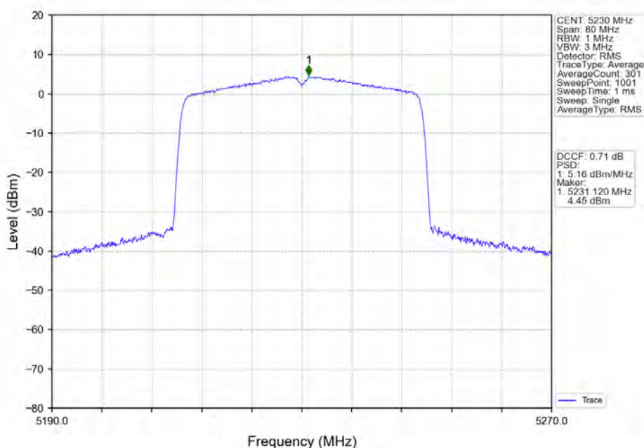
802.11ax(HE40)_HCH_5230MHz_RU484_Left_Ant2_NTNV
