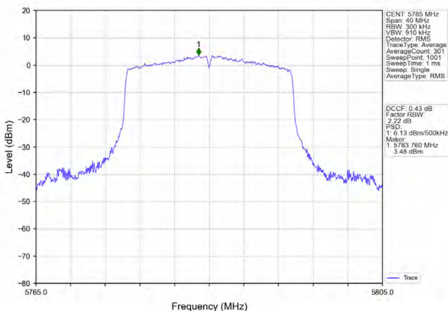
802.11ax(HE20)_MCH_5785MHz_RU242_Left_Ant2_NTNV
