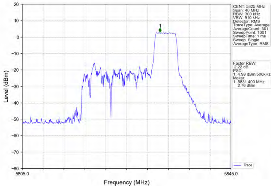
802.11ax(HE20)_HCH_5825MHz_RU52_Right_Ant1_NTNV
