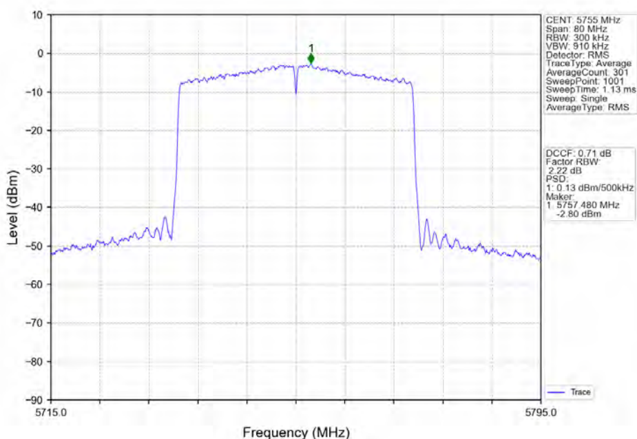
802.11ax(HE40)_LCH_5755MHz_RU484_Left_Ant2_NTNV
