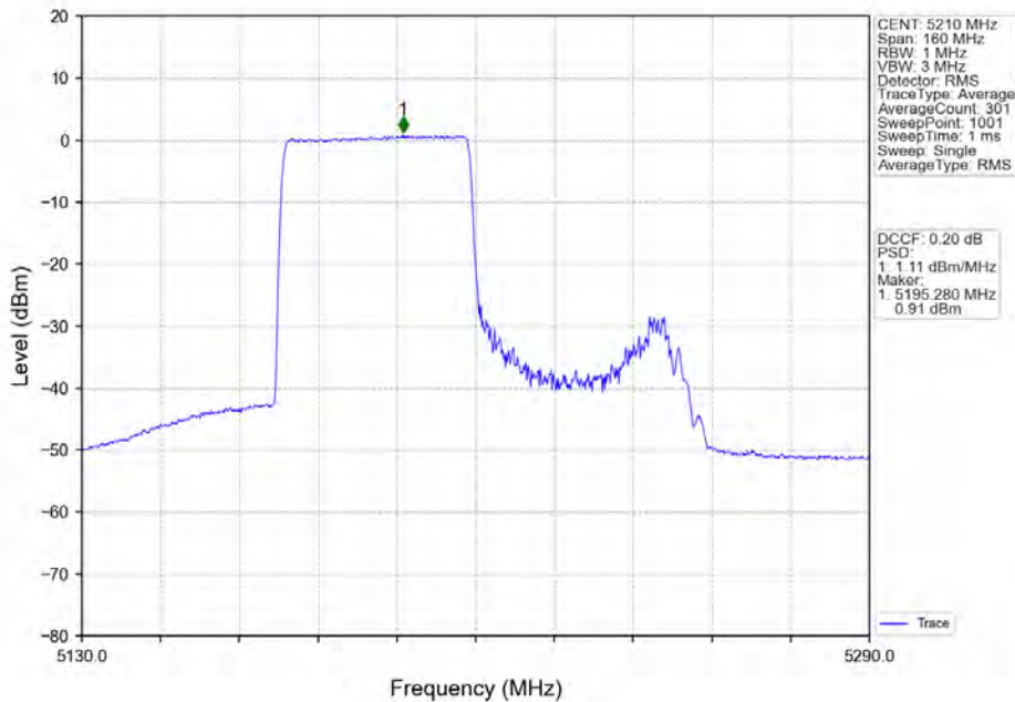
802.11ax(HE80)_MCH_5210MHz_RU484_Left_Ant2_NTNV
