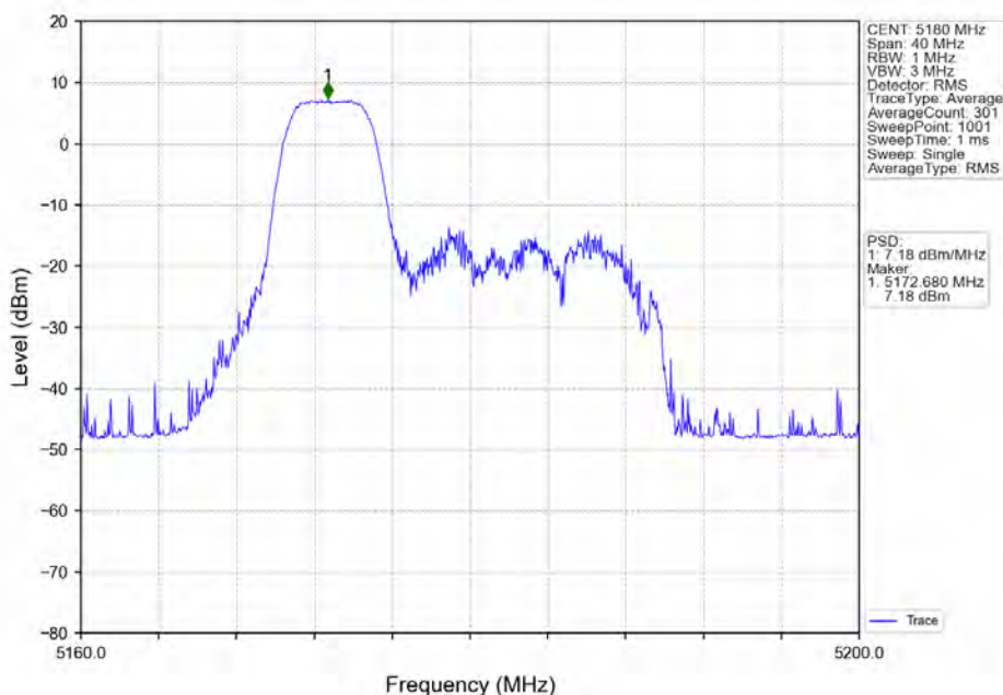
802.11ax(HE20)_LCH_5180MHz_RU52_Left_Ant1_NTNV
