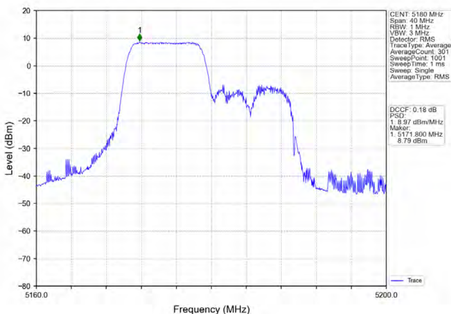
802.11ax(HE20)_LCH_5180MHz_RU106_Left_Ant2_NTNV
