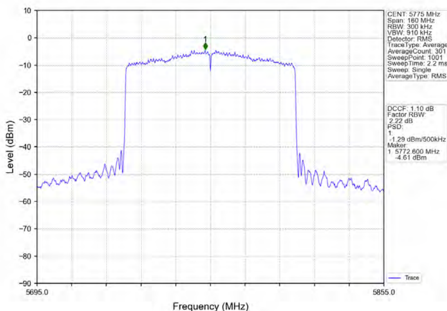
802.11ax(HE80)_MCH_5775MHz_RU996_Left_Ant1_NTNV
