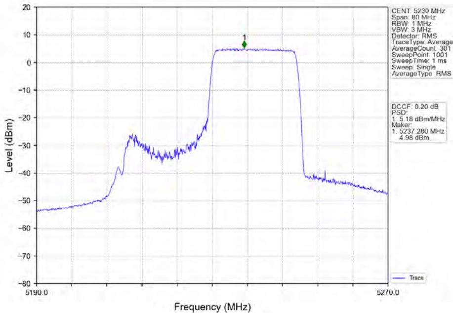
802.11ax(HE40) HCH_5230MHz_RU242_Right_Ant2_NTNV
