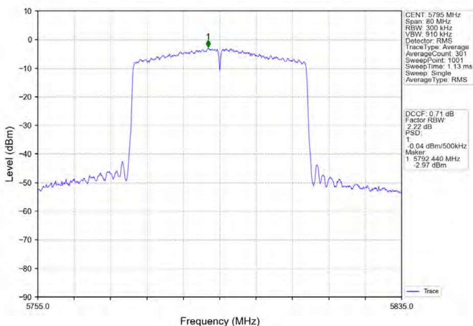
802.11ax(HE40)_HCH_5795MHz_RU484_Left_Ant2_NTNV
