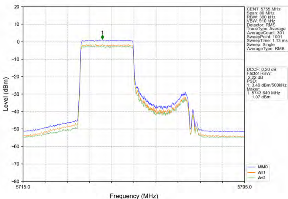
802.11ax(HE40) LCH_5755MHz_RU242_Left_MIMO_NTNV
