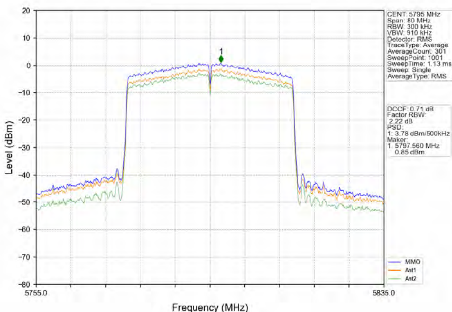
802.11ax(HE40) HCH_5795MHz_RU484_Left_MIMO_NTNV
