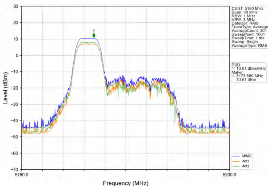
802.11ax(HE20)_LCH_5180MHz_RU52_Left MIMO_NTNV
