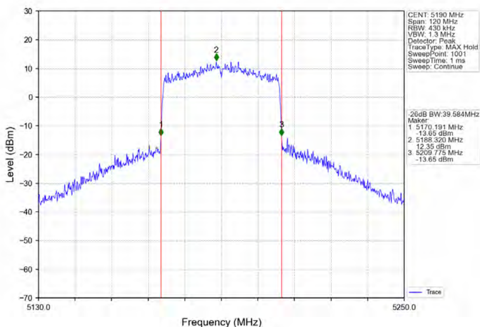
802.11ax(HE40)_LCH_5190MHz_RU484_Left_Ant2_NTNV
