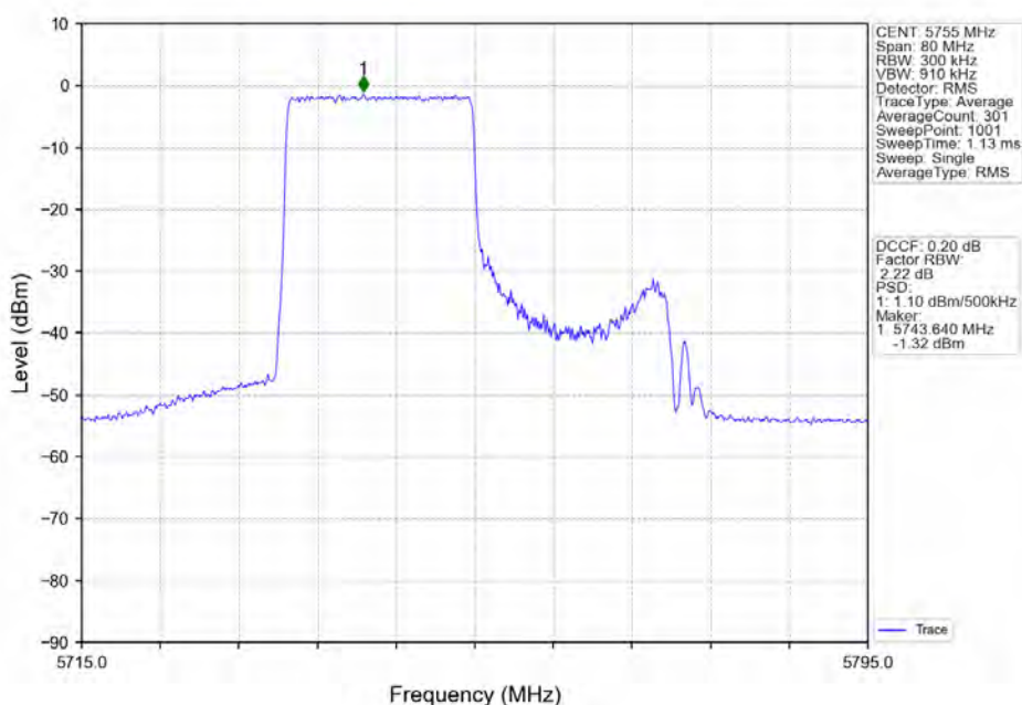
802.11ax(HE40)_LCH_5755MHz_RU242_Left_Ant1_NTNV
