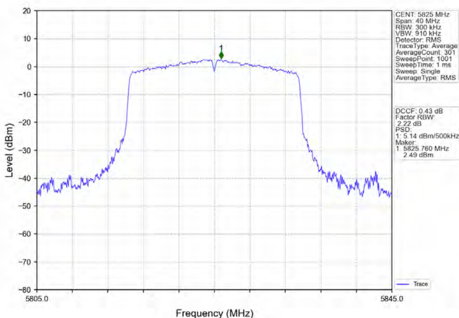
802.11ax(HE20)_HCH_5825MHz_RU242_Left_Ant2_NTNV
