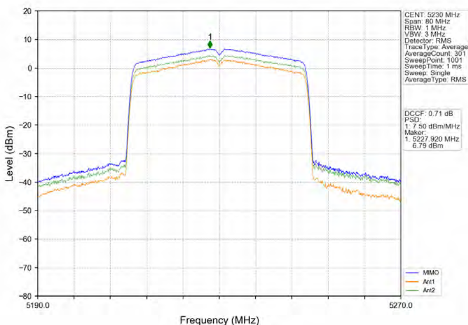
802.11ax(HE40)_HCH_5230MHz_RU484_Left_MIMO_NTNV
