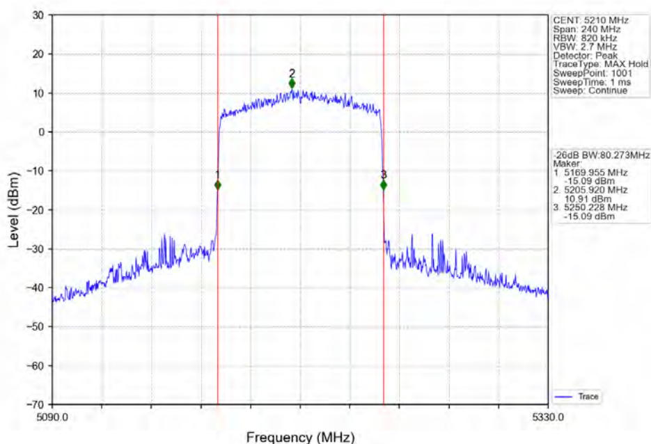
802.11ax(HE80)_MCH_5210MHz_RU996_Left_Ant2_NTNV
