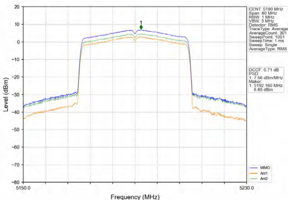
802.11ax(HE40) LCH_5190MHz_RU484_Left_MIMO_NTNV
