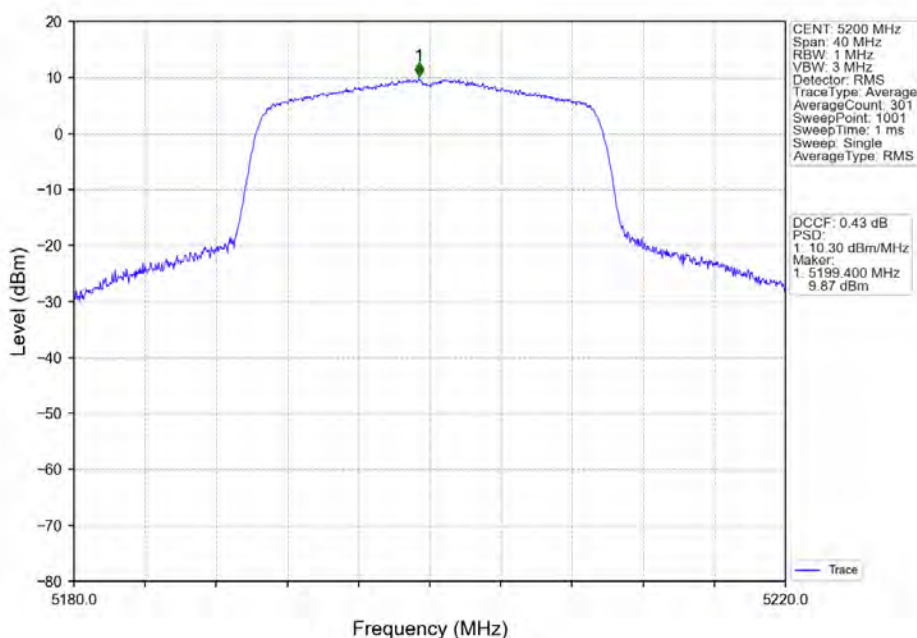
802.11ax(HE20)_MCH_5200MHz_RU242_Left_Ant2_NTNV
