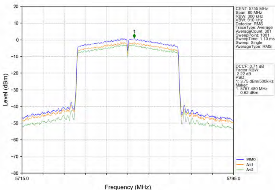
802.11ax(HE40) LCH_5755MHz_RU484_Left_MIMO_NTNV
