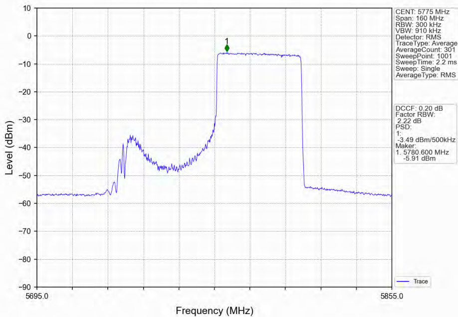
802.11ax(HE80)_MCH_5775MHz_RU484_Right_Ant2_NTNV
