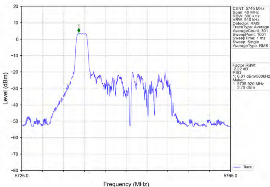
802.11ax(HE20)_LCH_5745MHz_RU26_Left_Ant2_NTNV
