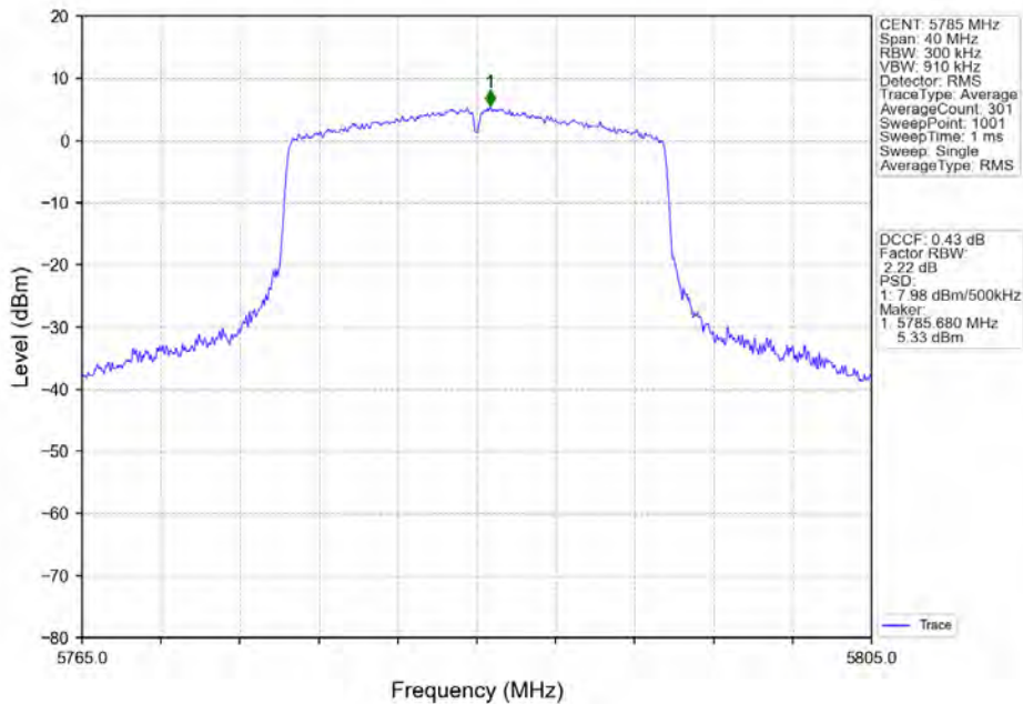
802.11ax(HE20)_MCH_5785MHz_RU242_Left_Ant1_NTNV
