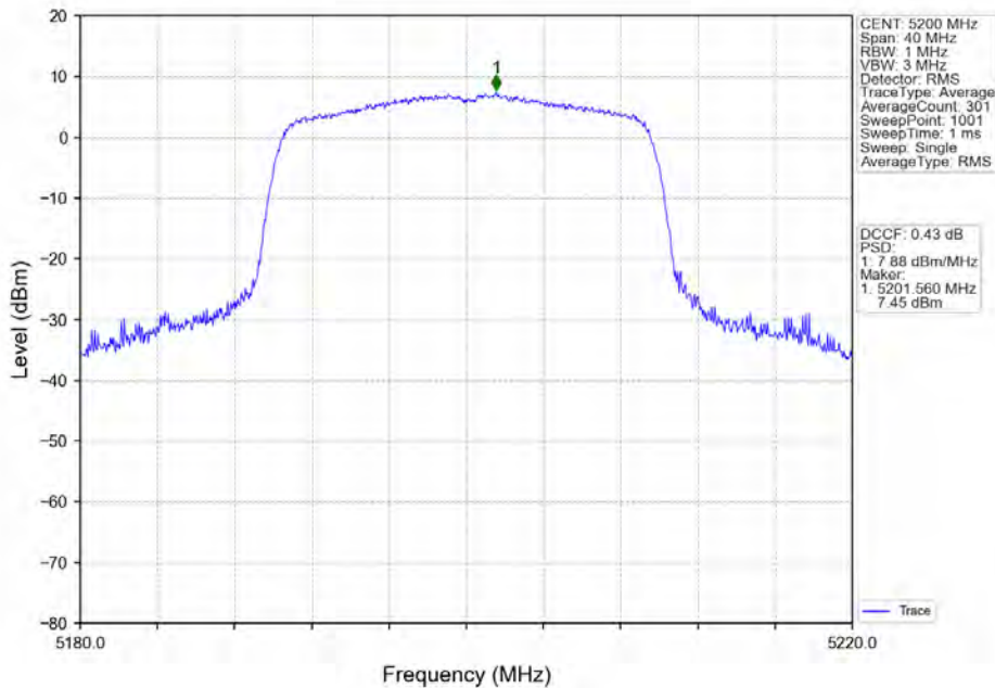
802.11ax(HE20)_MCH_5200MHz_RU242_Left_Ant1_NTNV
