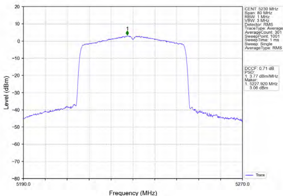
802.11ax(HE40)_HCH_5230MHz_RU484_Left_Ant1_NTNV
