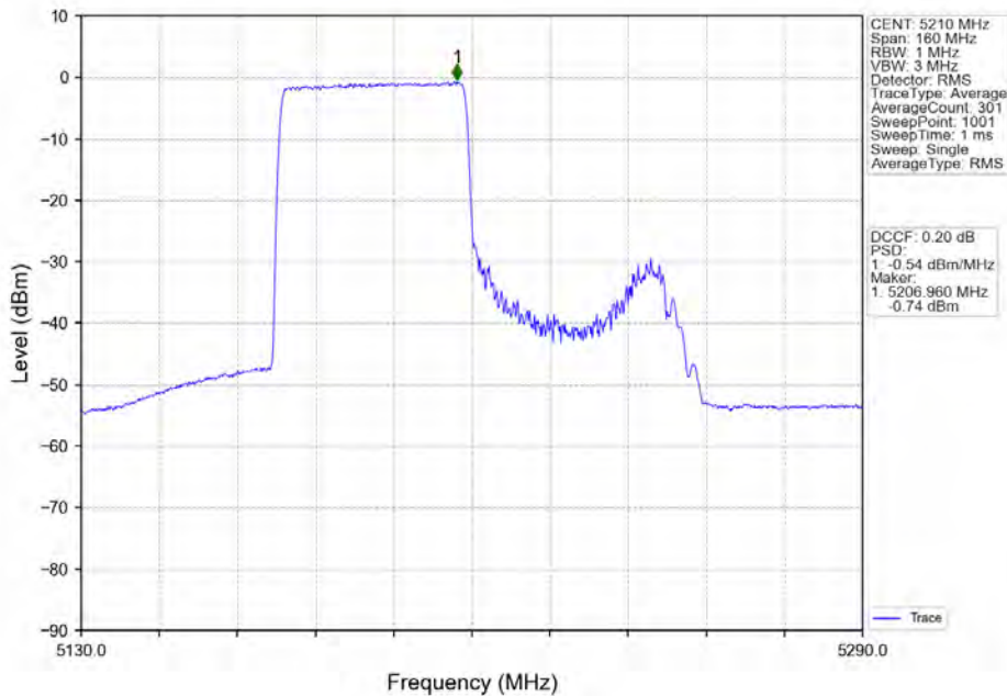
802.11ax(HE80)_MCH_5210MHz_RU484_Left_Ant1_NTNV
