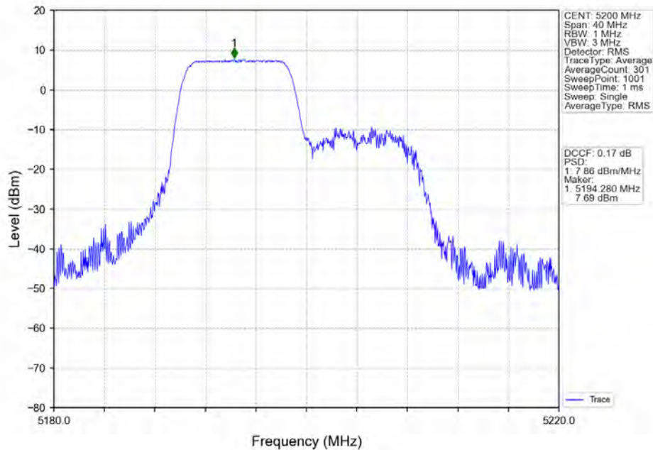
802.11ax(HE20)_MCH_5200MHz_RU106_Left_Ant1_NTNV
