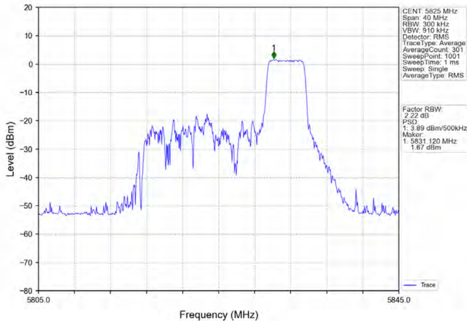
802.11ax(HE20)_HCH_5825MHz_RU52_Right_Ant2_NTNV
