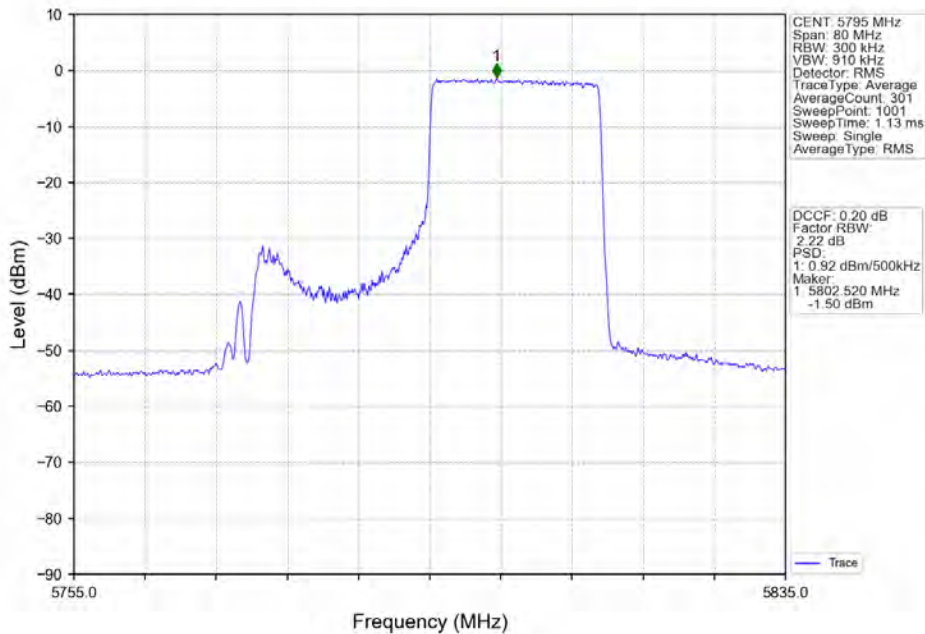
802.11ax(HE40) HCH_5795MHz_RU242_Right_Ant1_NTNV
