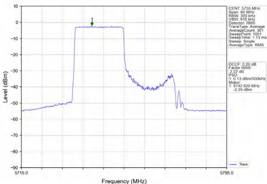
802.11ax(HE40)_LCH_5755MHz_RU242_Left_Ant2_NTNV
