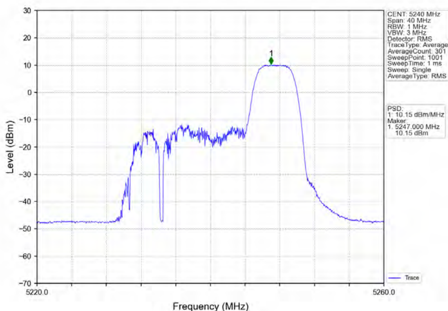
802.11ax(HE20)_HCH_5240MHz_RU52_Right_Ant2_NTNV
