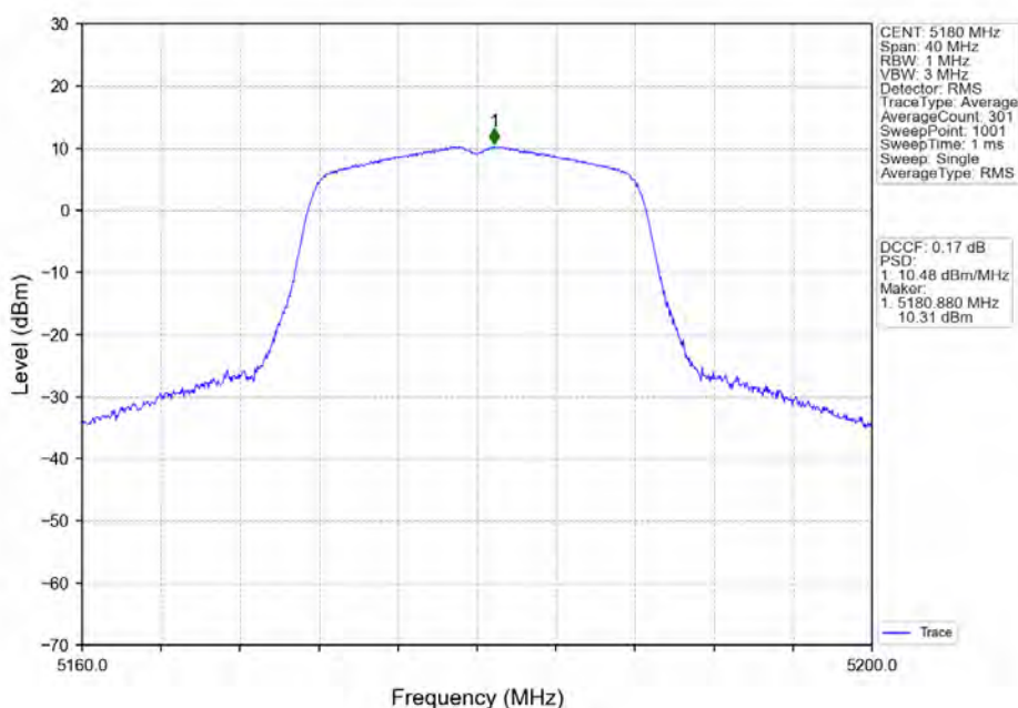
802.11a_LCH_5180MHz_Ant2_NTNV
