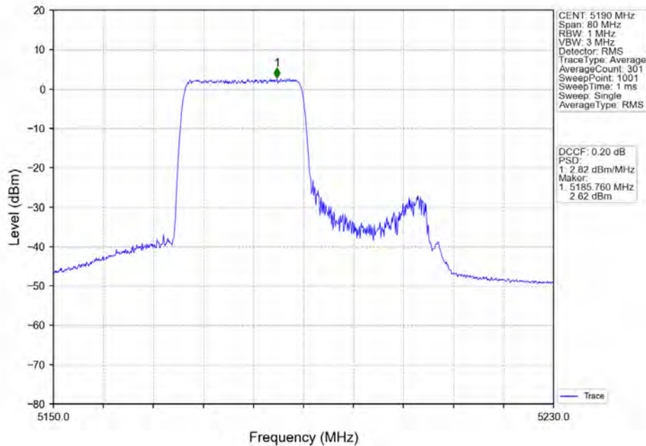
802.11ax(HE40)_LCH_5190MHz_RU242_Left_Ant2_NTNV
