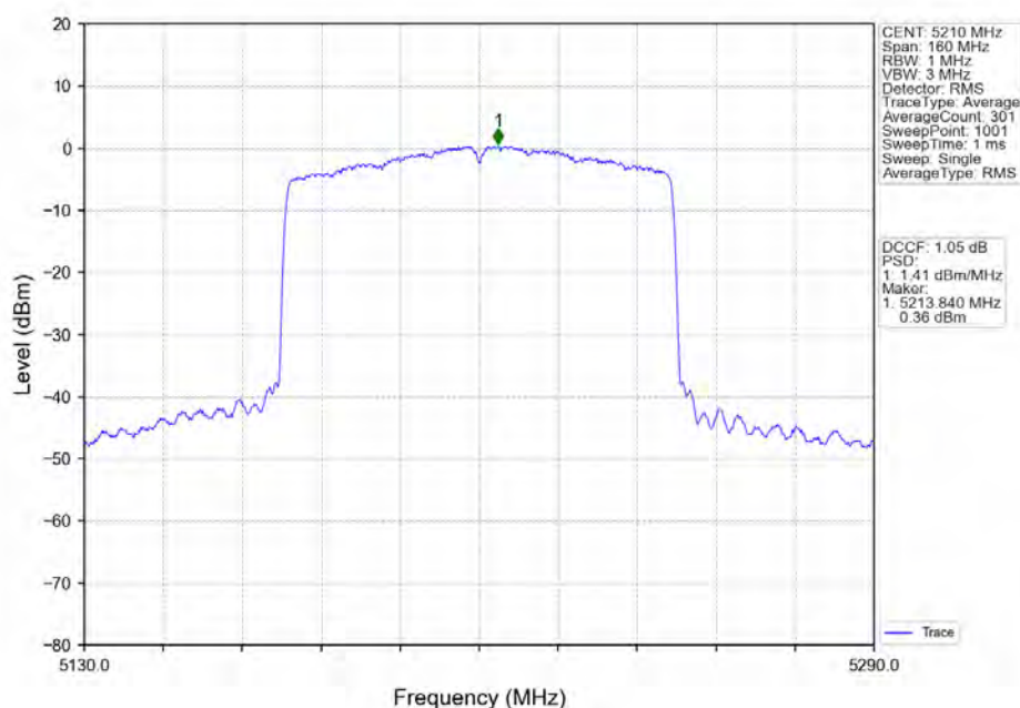
802.11ax(HE80)_MCH_5210MHz_RU996_Left_Ant2_NTNV
