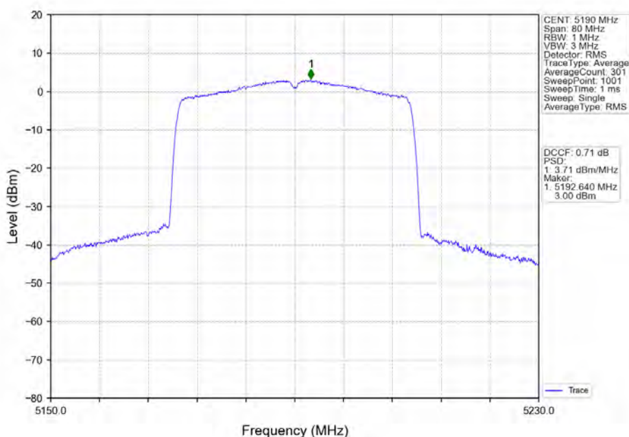
802.11ax(HE40)_LCH_5190MHz_RU484_Left_Ant1_NTNV
