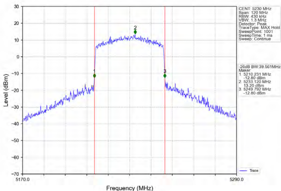
802.11ax(HE40)_HCH_5230MHz_RU484_Left_Ant2_NTNV
