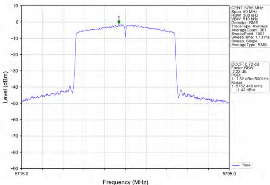
802.11ax(HE40)_LCH_5755MHz_RU484_Left_Ant1_NTNV
