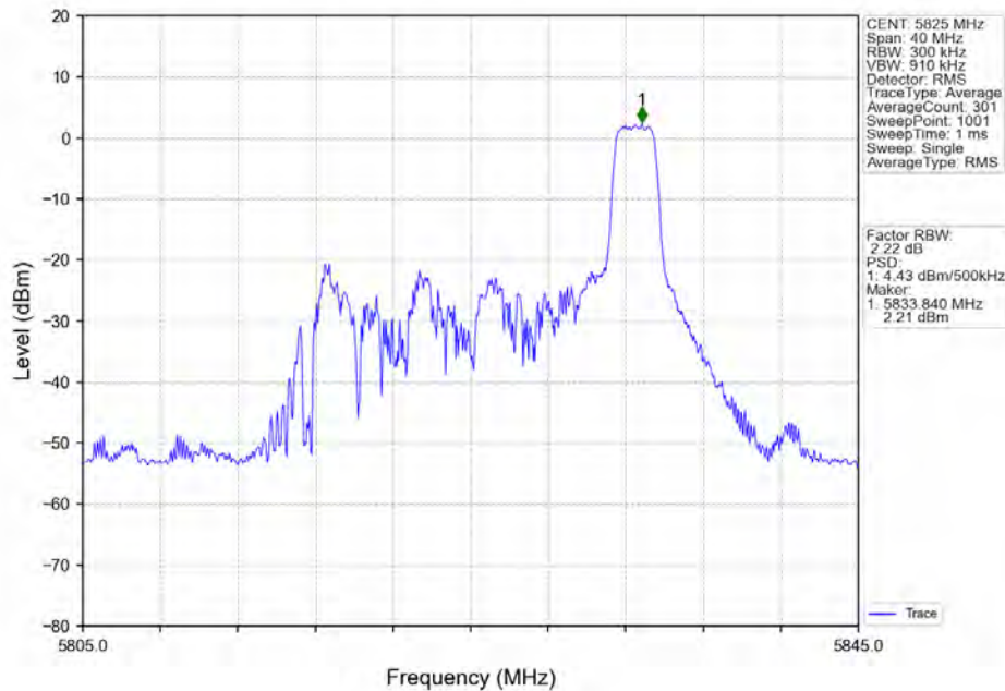
802.11ax(HE20)_HCH_5825MHz_RU26_Right_Ant2_NTNV
