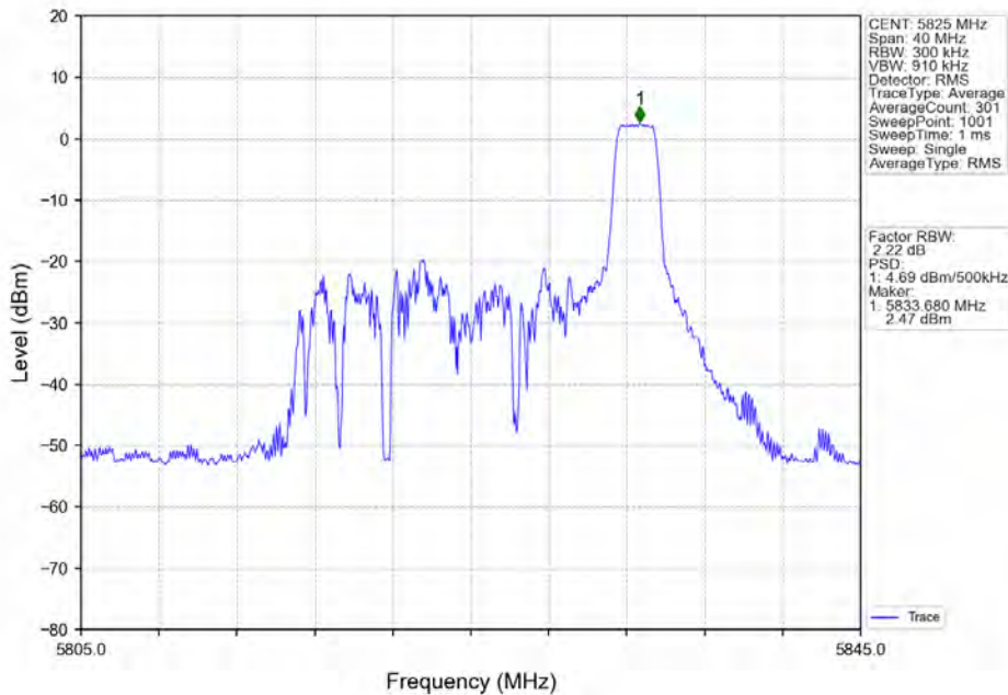
802.11ax(HE20)_HCH_5825MHz_RU26_Right_Ant1_NTNV
