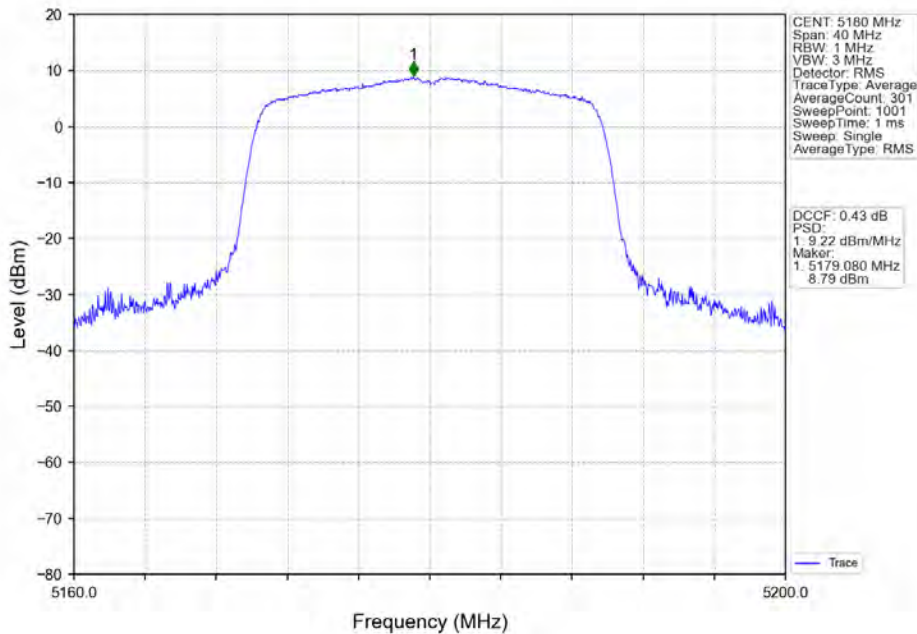
802.11ax(HE20)_LCH_5180MHz_RU242_Left_Ant2_NTNV
