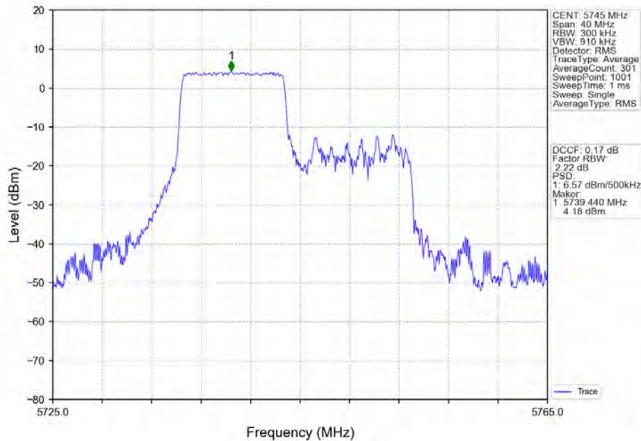
802.11ax(HE20)_LCH_5745MHz_RU106_Left_Ant1_NTNV
