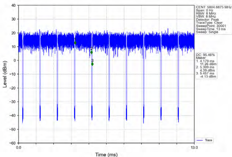
802.11ax(HE40) HCH_5795MHz_RU242_Right_Ant2_NTNV
