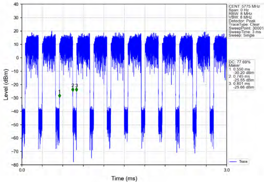
802.11ax(HE80)_MCH_5775MHz_RU996_Left_Ant1_NTNV
