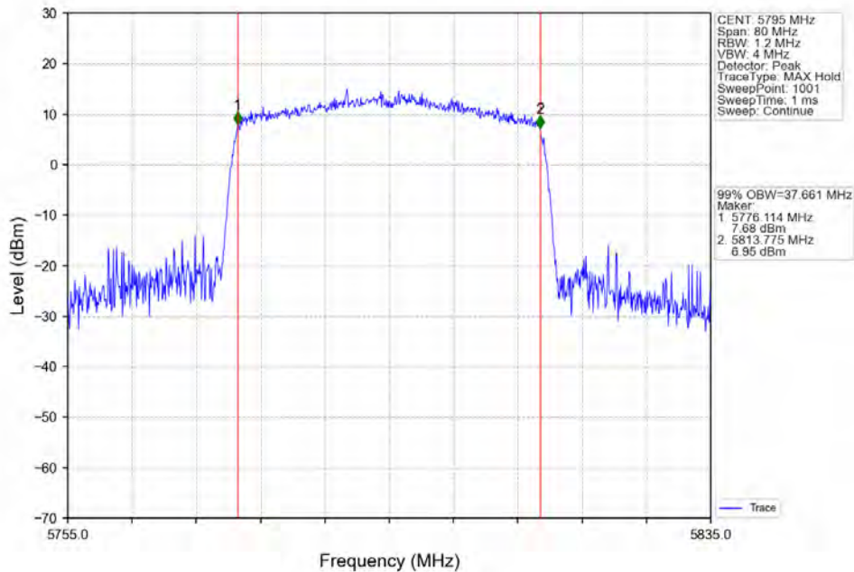
802.11ax(HE40)_HCH_5795MHz_RU484_Left_Ant2_NTNV
