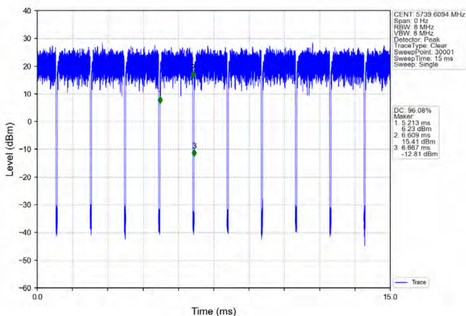
802.11ax(HE20)_LCH_5745MHz_RU106_Left_Ant1_NTNV
