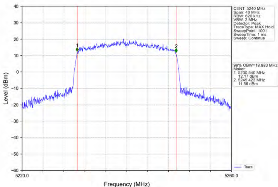
802.11ax(HE20)_HCH_5240MHz_RU242_Left_Ant2_NTNV
