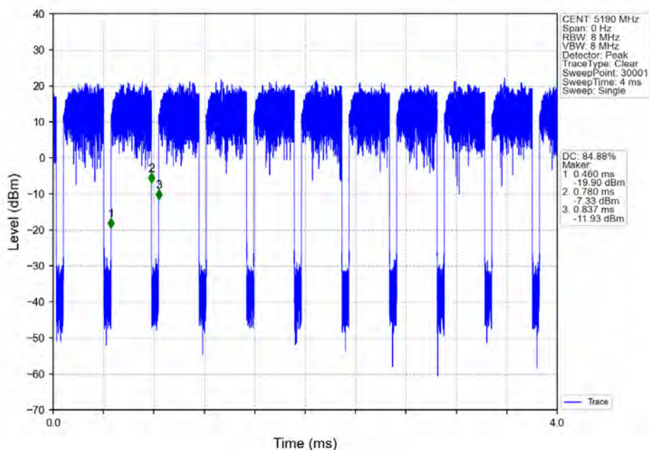
802.11ax(HE40)_LCH_5190MHz_RU484_Left_Ant1_NTNV
