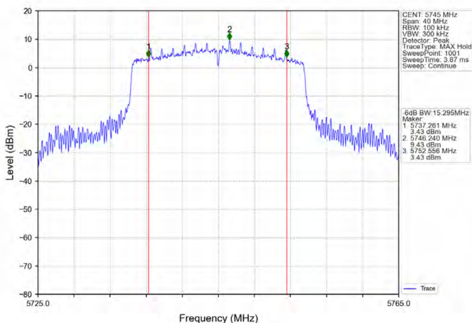
802.11ax(HE20)_LCH_5745MHz_RU242_Left_Ant2_NTNV
