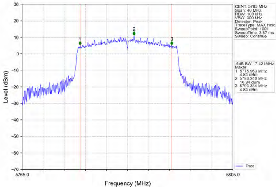
802.11ax(HE20)_MCH_5785MHz_RU242_Left_Ant1_NTNV
