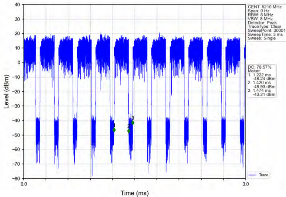
802.11ax(HE80)_MCH_5210MHz_RU996_Left_Ant2_NTNV
