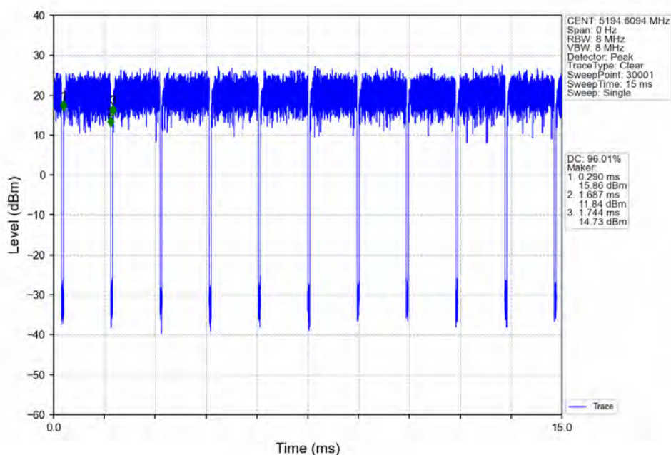
802.11ax(HE20)_MCH_5200MHz_RU106_Left_Ant2_NTNV
