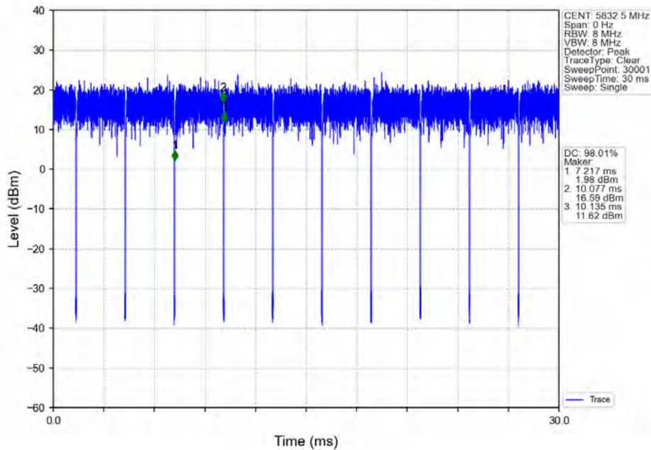
802.11ax(HE20)_HCH_5825MHz_RU52_Right_Ant2_NTNV
