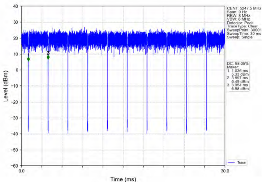
802.11ax(HE20)_HCH_5240MHz_RU52_Right_Ant2_NTNV
