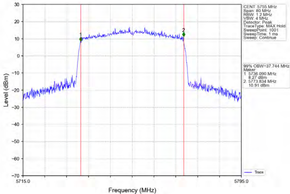
802.11ax(HE40)_LCH_5755MHz_RU484_Left_Ant1_NTNV
