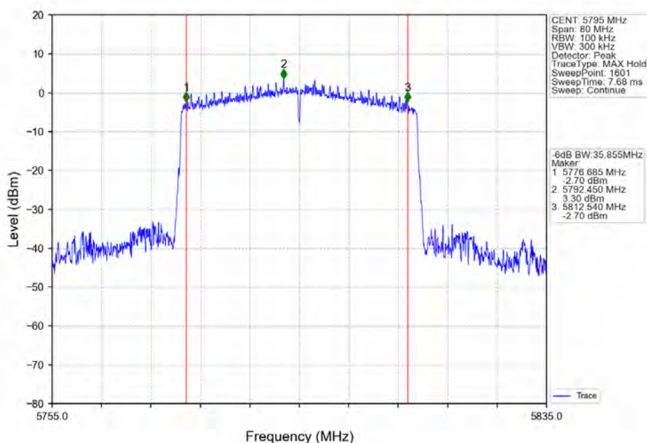
802.11ax(HE40)_HCH_5795MHz_RU484_Left_Ant2_NTNV
