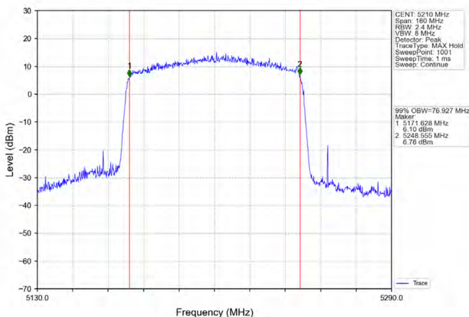
802.11ax(HE80)_MCH_5210MHz_RU996_Left_Ant1_NTNV
