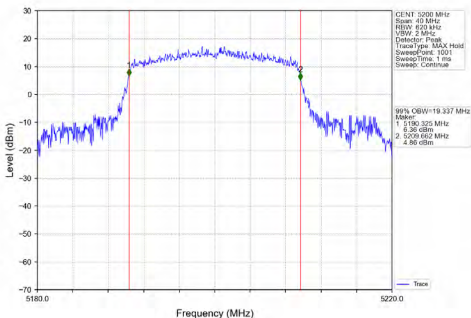
802.11ax(HE20)_MCH_5200MHz_RU242_Left_Ant1_NTNV
