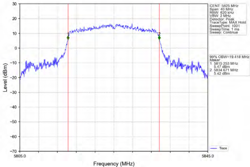
802.11ax(HE20)_HCH_5825MHz_RU242_Left_Ant2_NTNV
