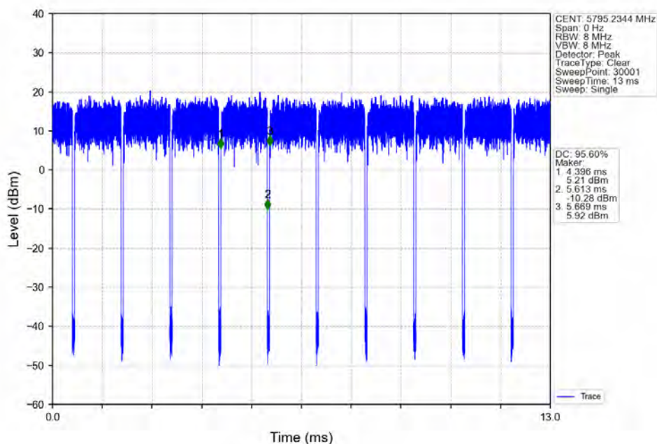
802.11ax(HE80)_MCH_5775MHz_RU484_Right_Ant1_NTNV
