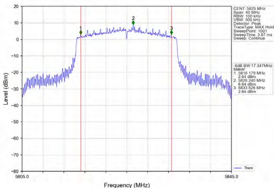
802.11ax(HE20)_HCH_5825MHz_RU242_Left_Ant2_NTNV
