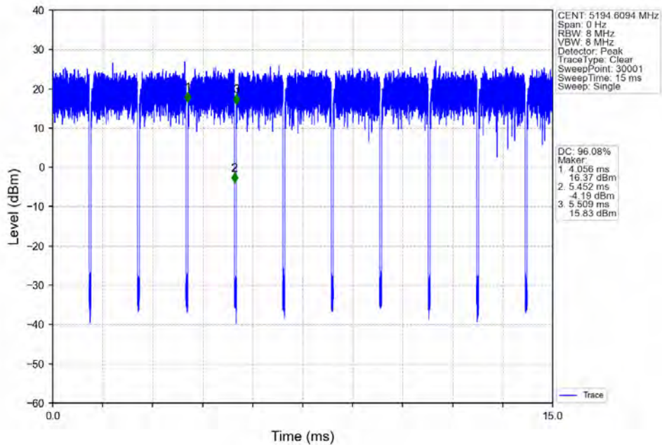
802.11ax(HE20)_MCH_5200MHz_RU106_Left_Ant1_NTNV
