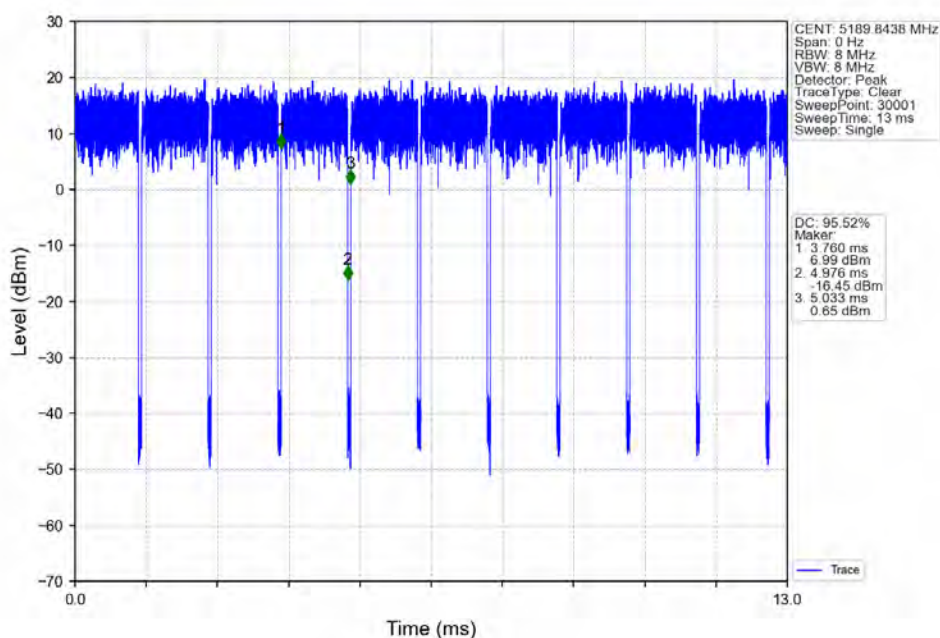
802.11ax(HE80)_MCH_5210MHz_RU484_Left_Ant2_NTNV
