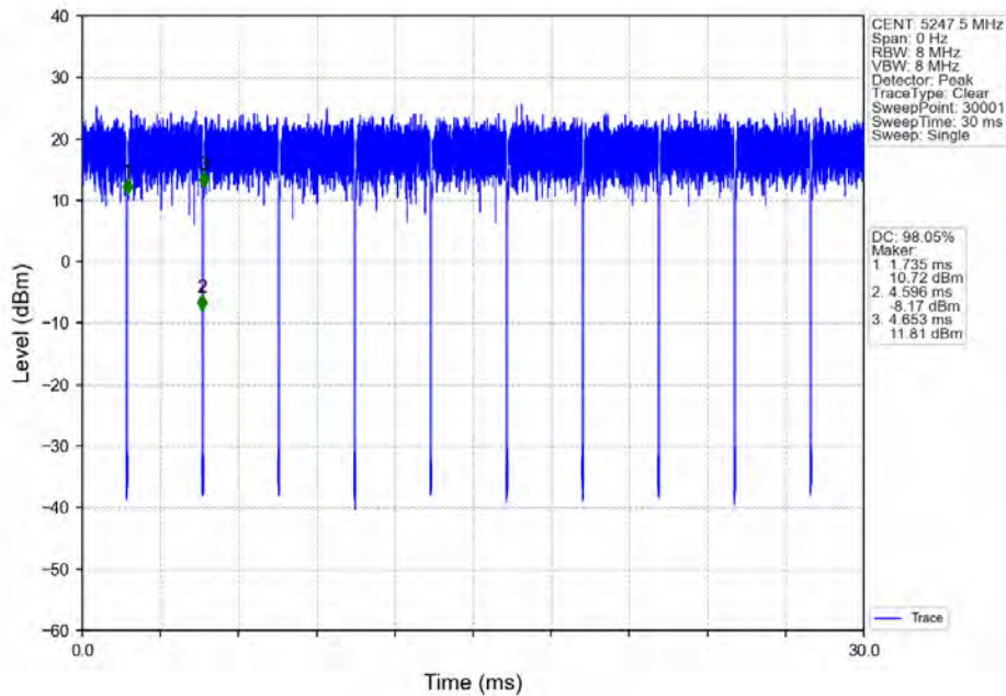
802.11ax(HE20)_HCH_5240MHz_RU52_Right_Ant1_NTNV
