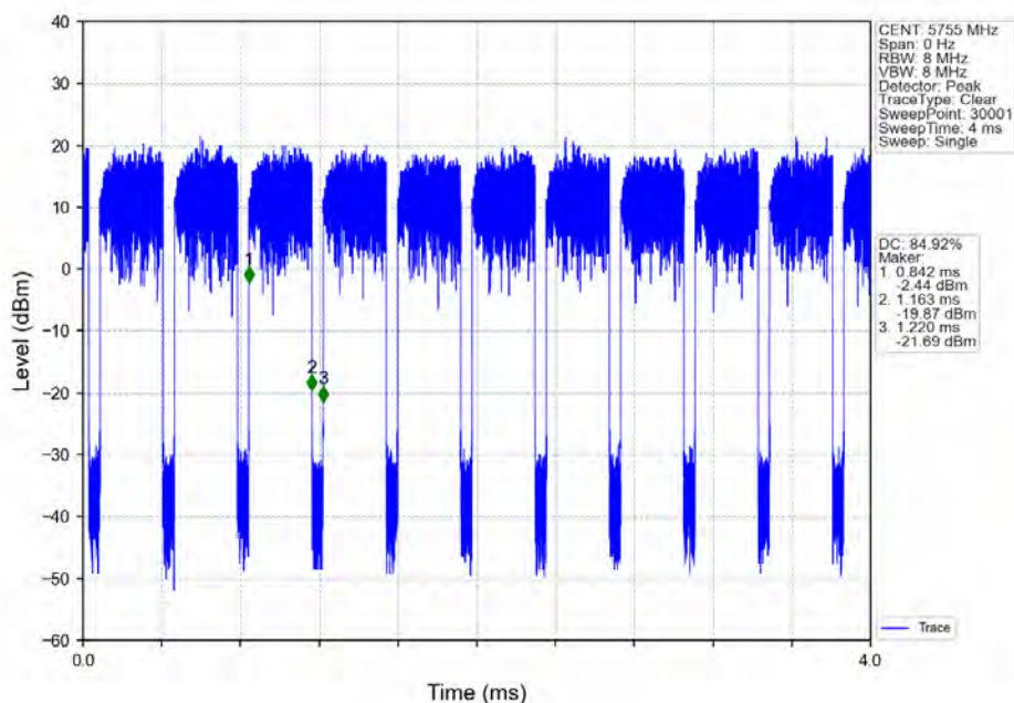
802.11ax(HE40)_LCH_5755MHz_RU484_Left_Ant2_NTNV
