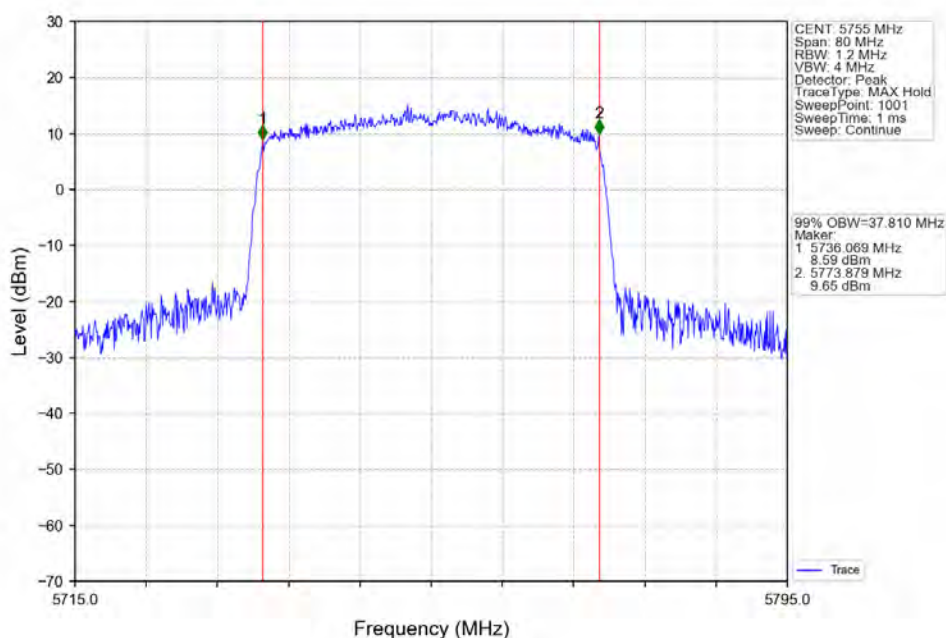
802.11ax(HE40)_LCH_5755MHz_RU484_Left_Ant2_NTNV
