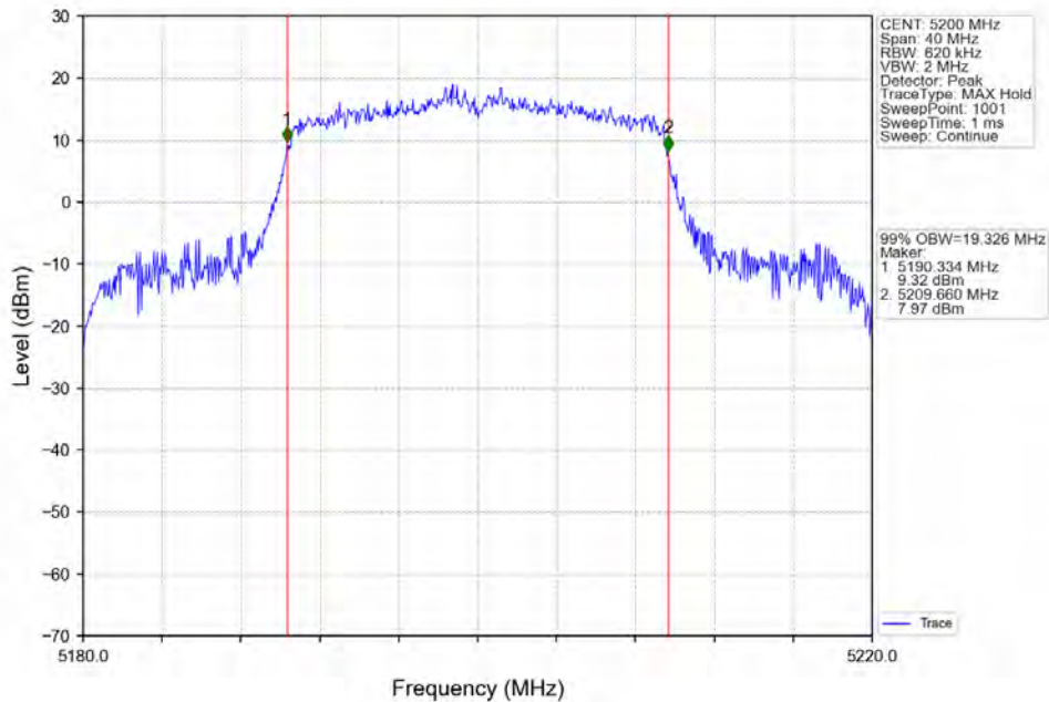
802.11ax(HE20)_MCH_5200MHz_RU242_Left_Ant2_NTNV
