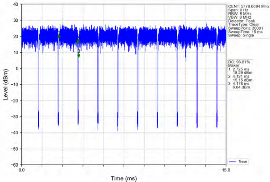
802.11ax(HE20)_MCH_5785MHz_RU106_Left_Ant1_NTNV
