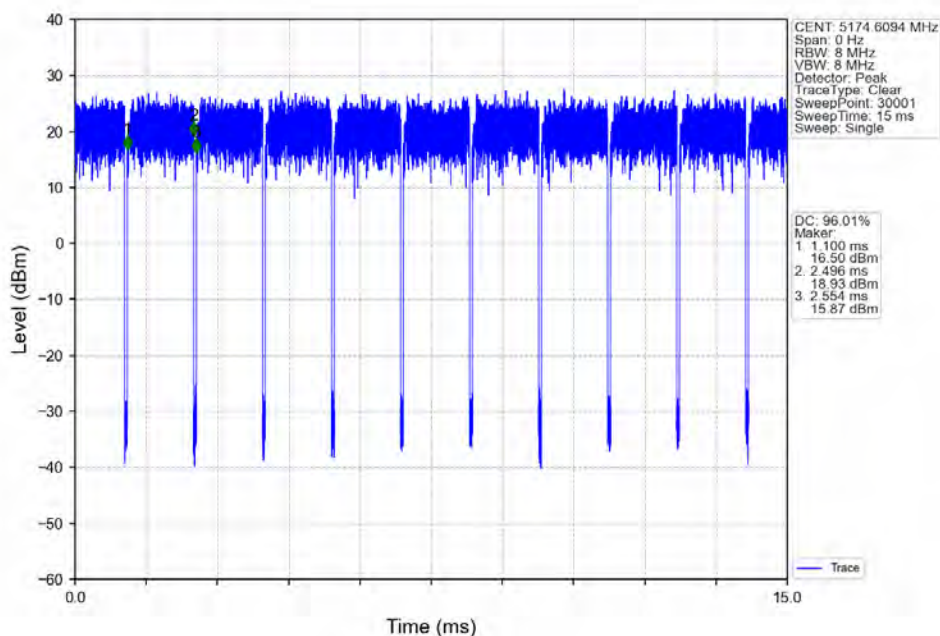
802.11ax(HE20)_LCH_5180MHz_RU106_Left_Ant2_NTNV
