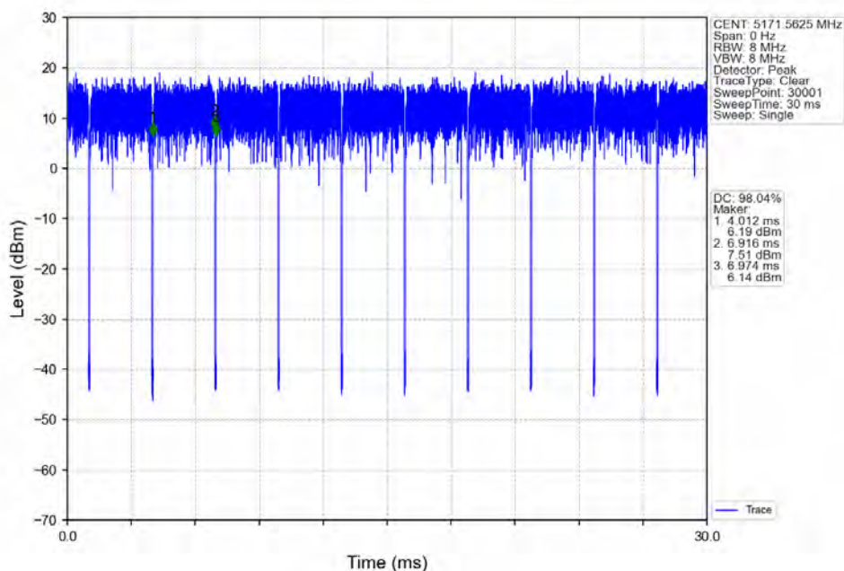
802.11ax(HE20)_LCH_5180MHz_RU26_Left_Ant2_NTNV
