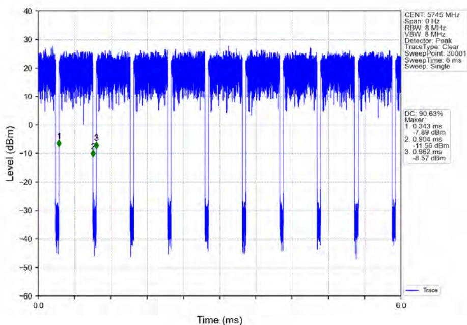
802.11ax(HE20)_LCH_5745MHz_RU242_Left_Ant1_NTNV
