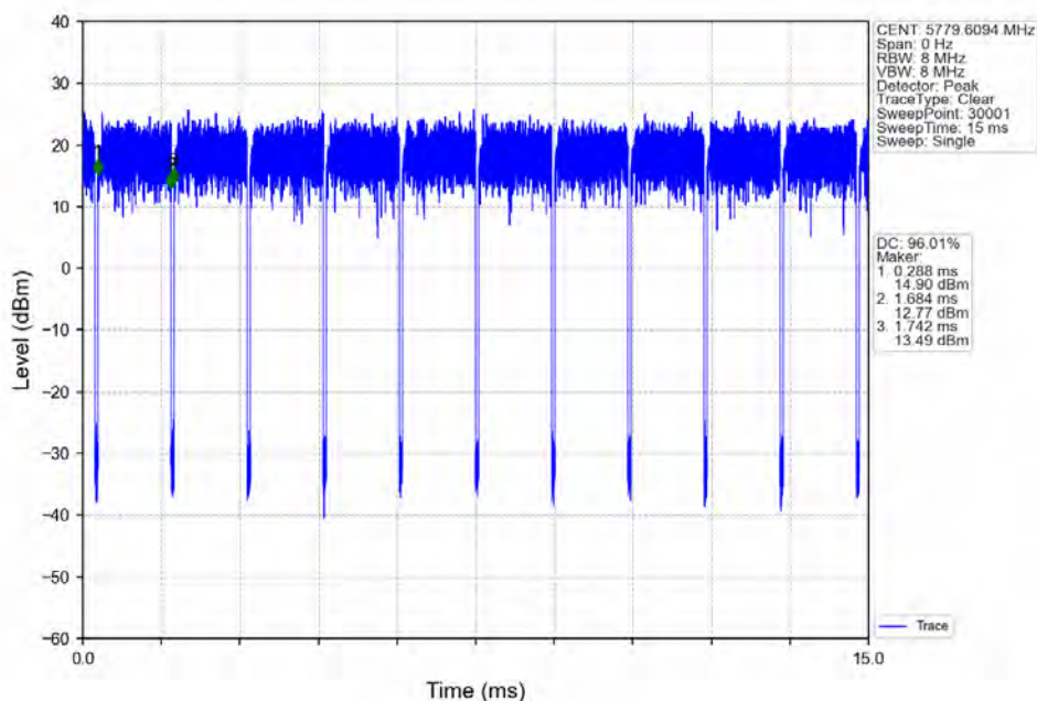
802.11ax(HE20)_MCH_5785MHz_RU106_Left_Ant2_NTNV
