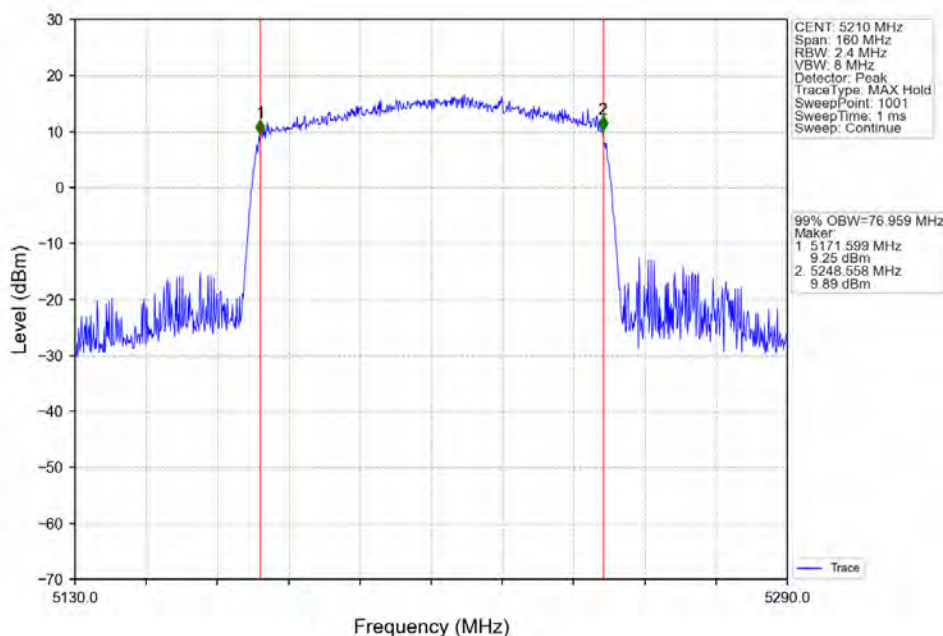
802.11ax(HE80)_MCH_5210MHz_RU996_Left_Ant2_NTNV
