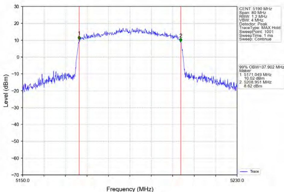
802.11ax(HE40)_LCH_5190MHz_RU484_Left_Ant2_NTNV
