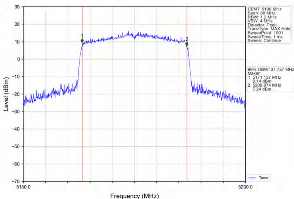
802.11ax(HE40)_LCH_5190MHz_RU484_Left_Ant1_NTNV
