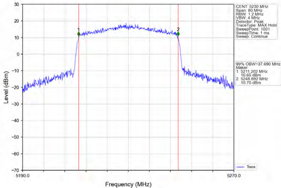
802.11ax(HE40)_HCH_5230MHz_RU484_Left_Ant2_NTNV
