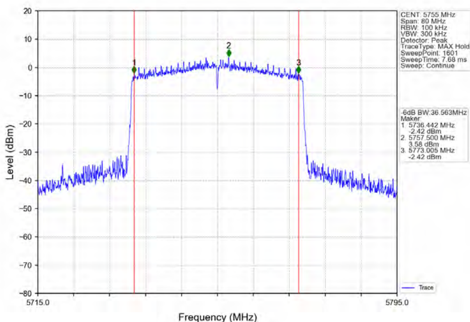
802.11ax(HE40)_LCH_5755MHz_RU484_Left_Ant2_NTNV
