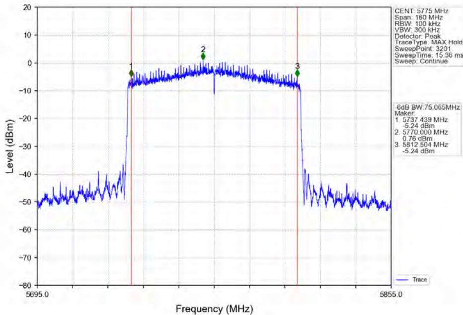
802.11ax(HE80)_MCH_5775MHz_RU996_Left_Ant2_NTNV
