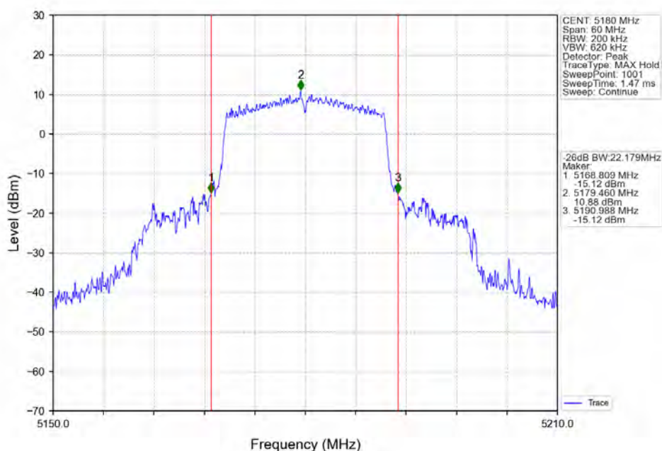
802.11ax(HE20)_LCH_5180MHz_RU242_Left_Ant1_NTNV
