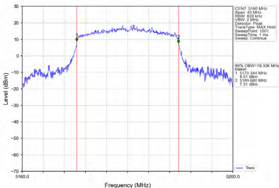
802.11ax(HE20)_LCH_5180MHz_RU242_Left_Ant2_NTNV
