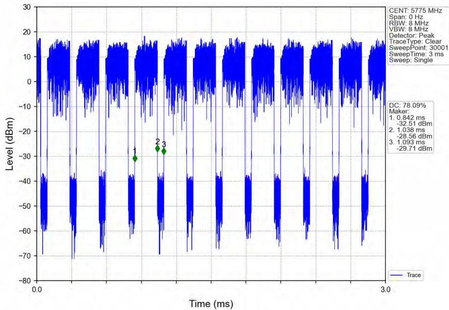
802.11ax(HE80)_MCH_5775MHz_RU996_Left_Ant2_NTNV
