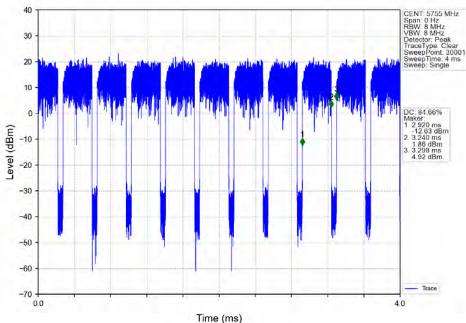
802.11ax(HE40)_LCH_5755MHz_RU484_Left_Ant1_NTNV
