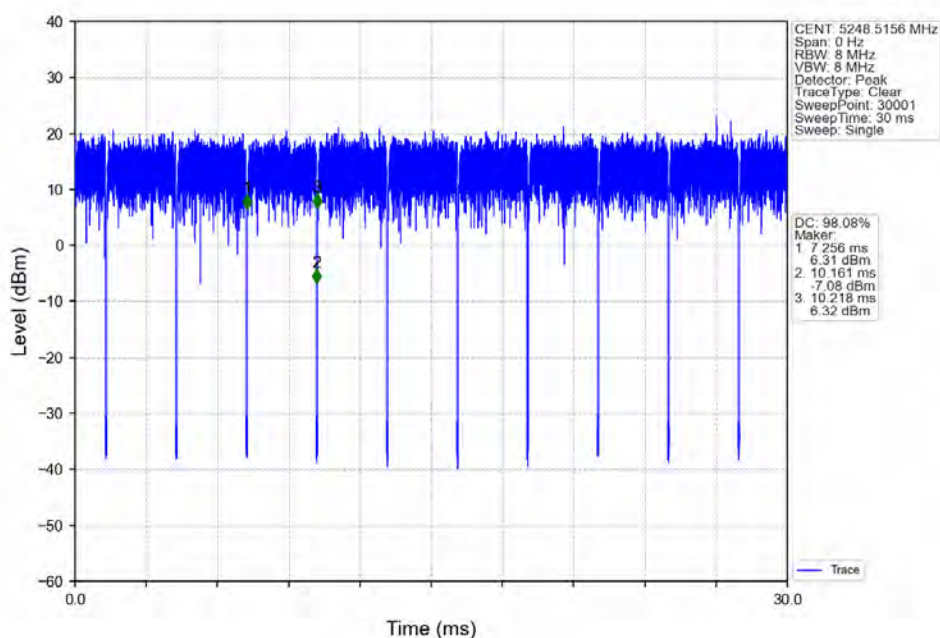
802.11ax(HE20)_HCH_5240MHz_RU26_Right_Ant1_NTNV
