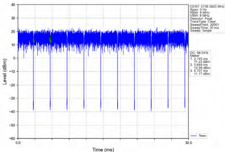
802.11ax(HE20)_LCH_5745MHz_RU26_Left_Ant1_NTNV
