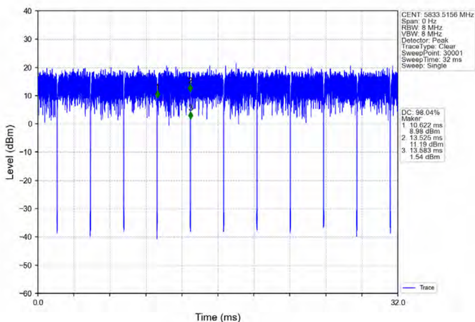
802.11ax(HE20)_HCH_5825MHz_RU26_Right_Ant1_NTNV
