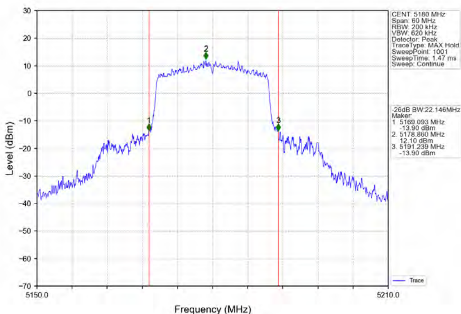
802.11ax(HE20)_LCH_5180MHz_RU242_Left_Ant2_NTNV
