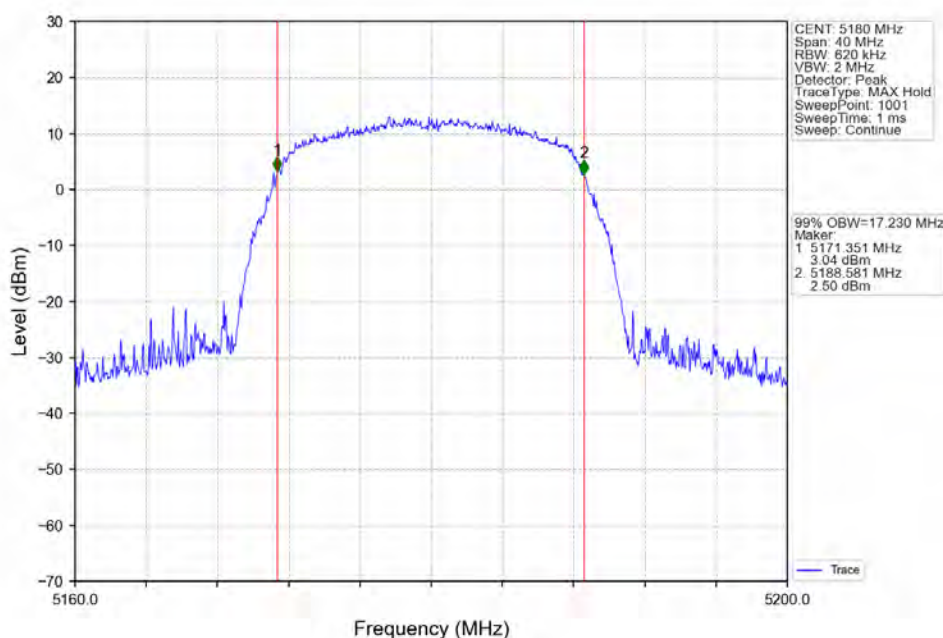
802.11a_LCH_5180MHz_Ant2_NTNV
