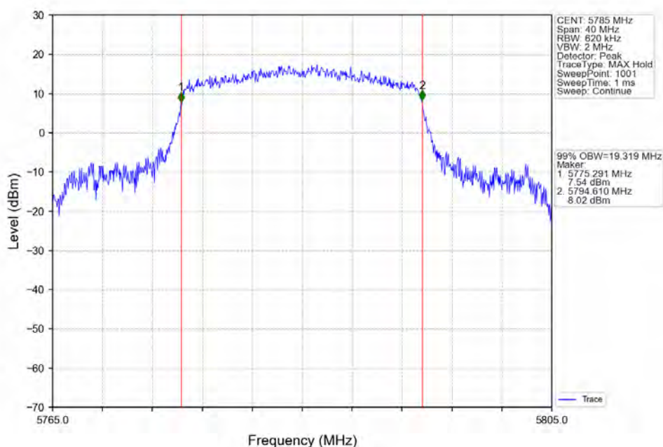
802.11ax(HE20)_MCH_5785MHz_RU242_Left_Ant2_NTNV
