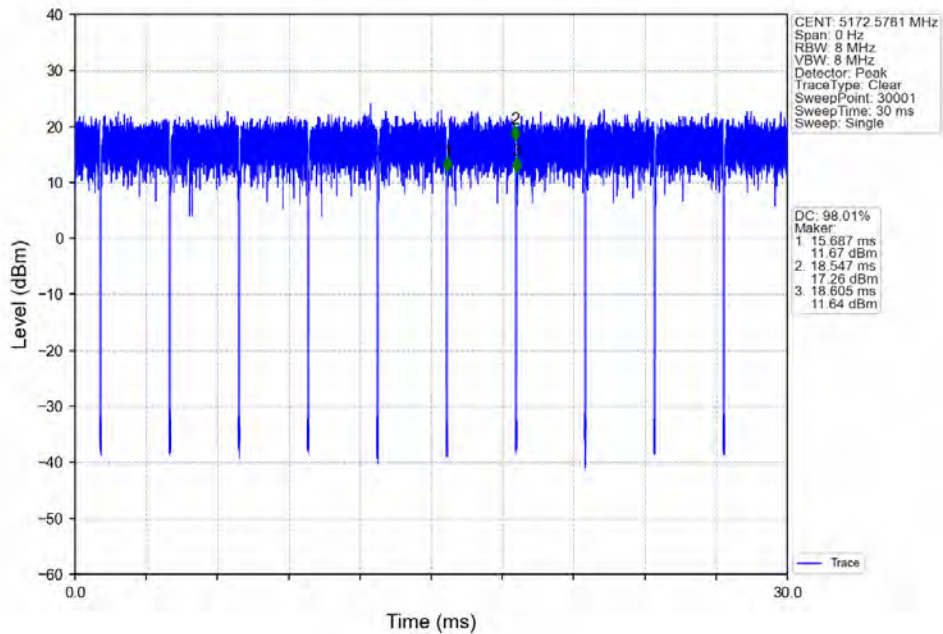
802.11ax(HE20)_LCH_5180MHz_RU52_Left_Ant1_NTNV
