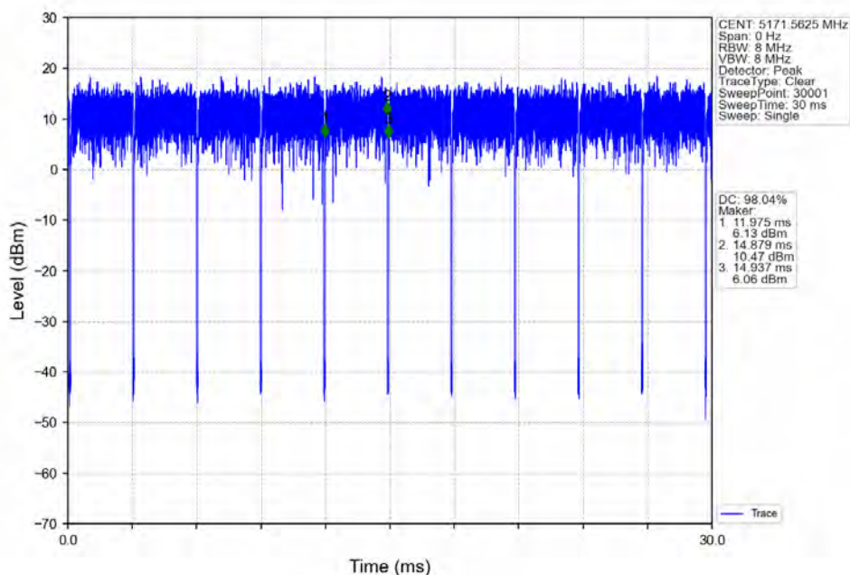
802.11ax(HE20)_LCH_5180MHz_RU26_Left_Ant1_NTNV
