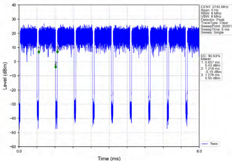
802.11ax(HE20)_LCH_5745MHz_RU242_Left_Ant2_NTNV
