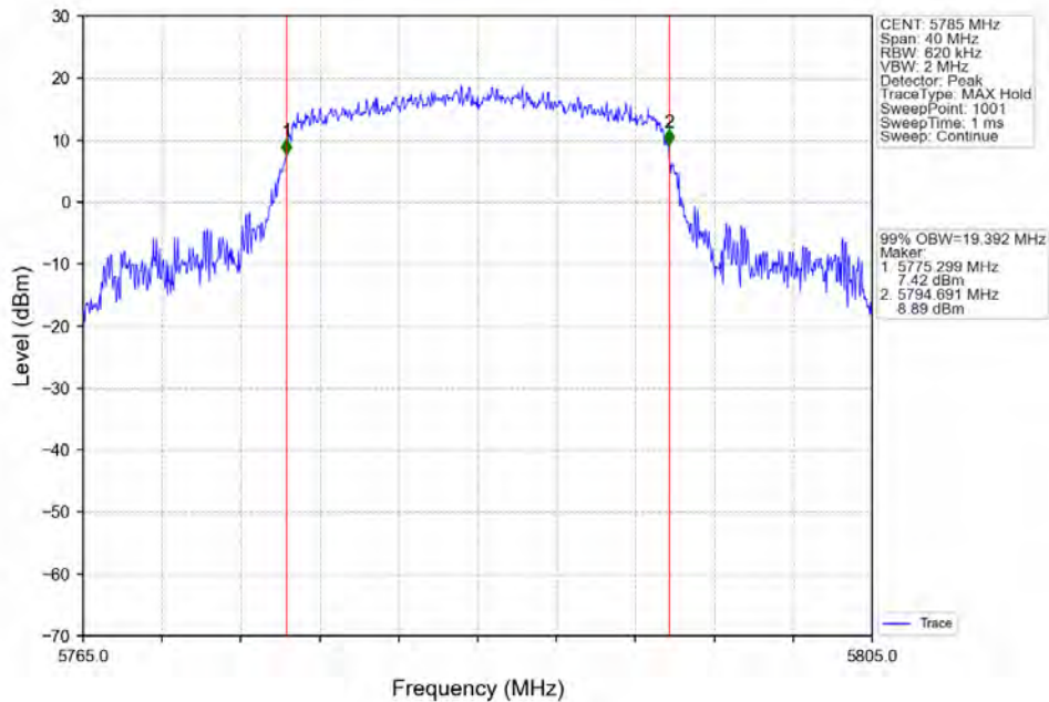
802.11ax(HE20)_MCH_5785MHz_RU242_Left_Ant1_NTNV
