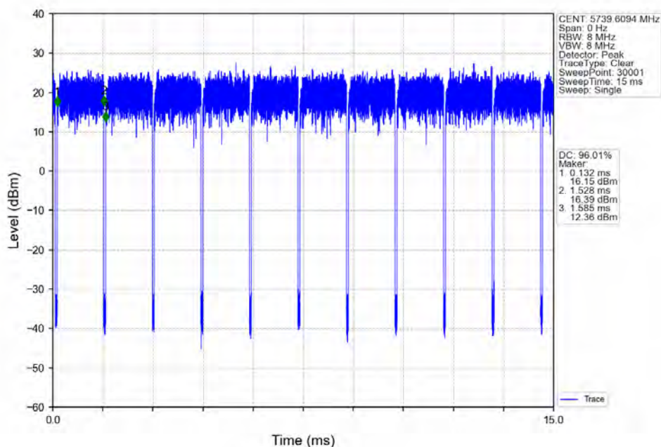
802.11ax(HE20)_LCH_5745MHz_RU106_Left_Ant2_NTNV
