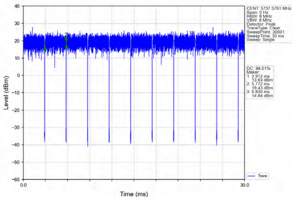
802.11ax(HE20)_LCH_5745MHz_RU52_Left_Ant1_NTNV
