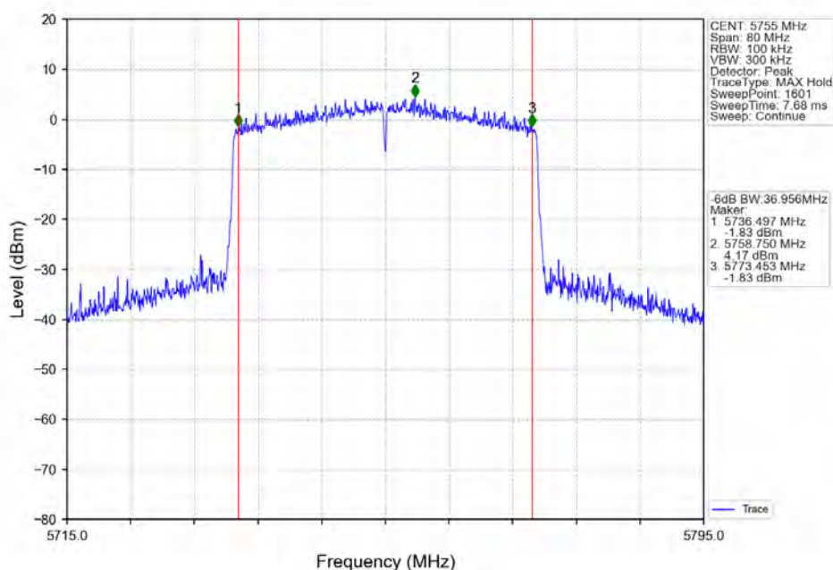
802.11ax(HE40)_LCH_5755MHz_RU484_Left_Ant1_NTNV
