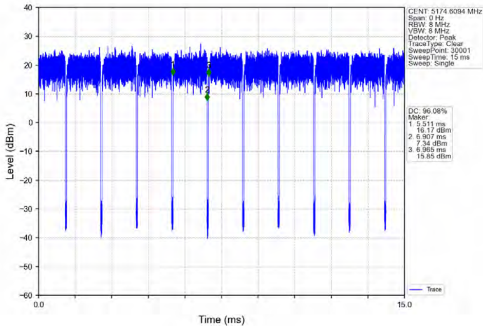
802.11ax(HE20)_LCH_5180MHz_RU106_Left_Ant1_NTNV
