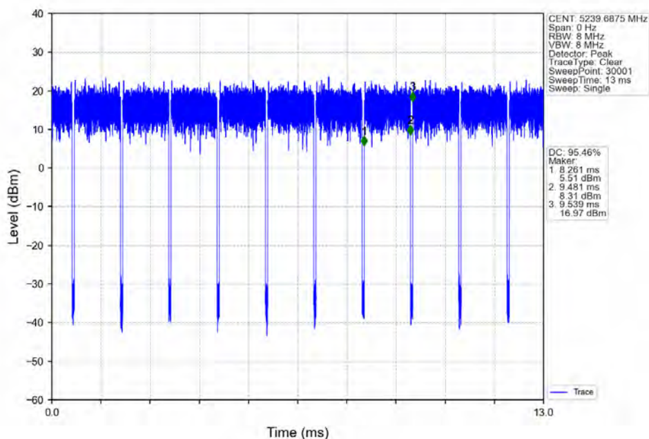
802.11ax(HE40)_HCH_5230MHz_RU242_Right_Ant1_NTNV
