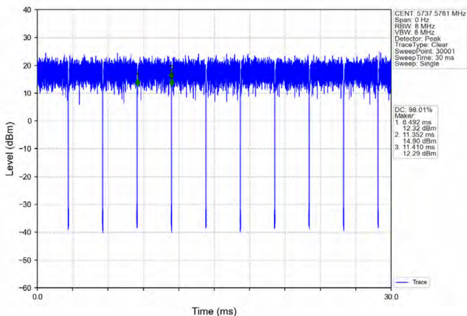
802.11ax(HE20)_LCH_5745MHz_RU52_Left_Ant2_NTNV
