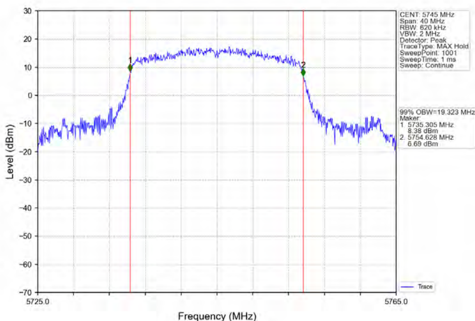
802.11ax(HE20)_LCH_5745MHz_RU242_Left_Ant2_NTNV
