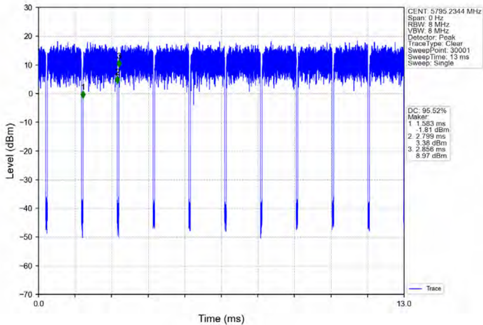
802.11ax(HE80)_MCH_5775MHz_RU484_Right_Ant2_NTNV
