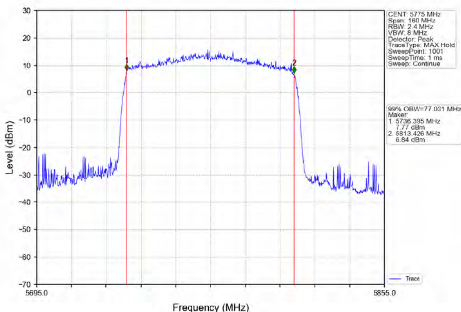
802.11ax(HE80)_MCH_5775MHz_RU996_Left_Ant2_NTNV
