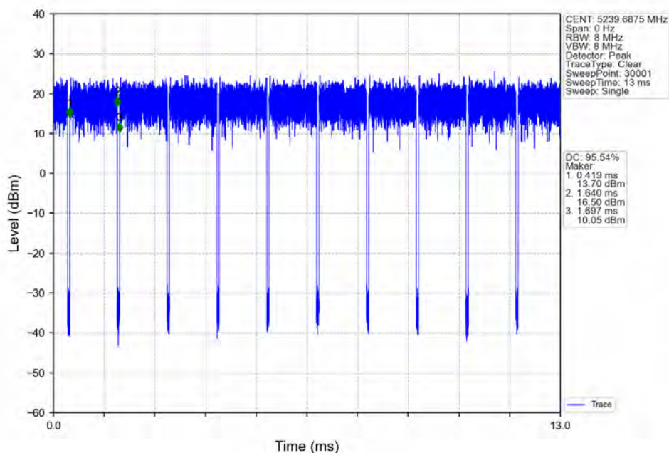
802.11ax(HE40)_HCH_5230MHz_RU242_Right_Ant2_NTNV
